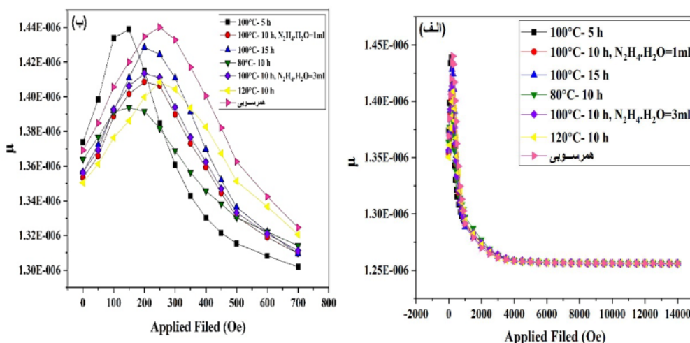
شکل ۹ نمودار نفوذپذیری مغناطیسی نانوذرات \text{FeNi}_3 تهیه شده به روش‌های گرمایی و هم‌رسوبی.
