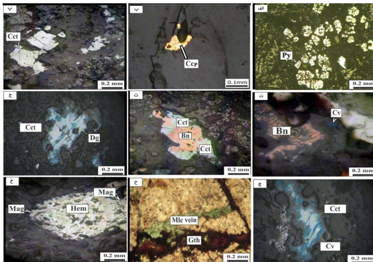
شکل ۶ تصاویر نوری بازتابی از الف) کانی پیریت (Py) در زمینه سنگ میزبان، ب) کالکوپیریت (Ccp)، پ) کالکوسیت (Cet)، ت) حضور کوولیت (Cv) در درزه‌ها و لبه کانه ایدایت، ث) جانشینی برنیت (Bn) با کالکوسیت، ج) جانشینی کالکوسیت با دیژنیت (Dg)، چ) جانشینی کالکوسیت با کوولیت، ح) رگه‌های گوئیتیت (Gth) و مالاکیت (Mlc)، خ) جانشینی مگنتیت (Mag) با هماتیت (Hem) در فرآیند مارتیتی شدن (مخفف کانی‌ها برگرفته از مرجع [۲۳]).
