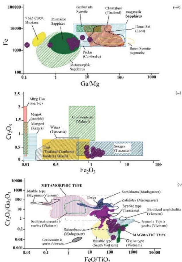
شکل ۶ نمودارهای رسم شده بر اساس داده‌های تجزیه شیمیایی بلورهای کروندوم خاکی به روش‌های XRF و ICP-MS: (الف) نمودار آهن (Fe) نسبت به Ga/Mg . نمودار پایه برگرفته از مراجع [۳۷، ۳۹، ۴۰] است، (ب) نمودار Cr_2O_3 نسبت به Fe_2O_3 که انواع ذخایر مختلف آفریقا را نشان می‌دهد. نمودار پایه برگرفته از مراجع [۲۲، ۳۶، ۴۱-۴۴] است.
