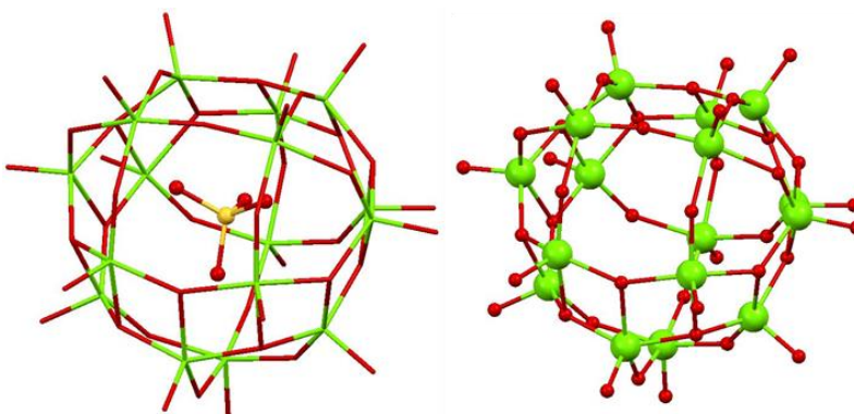
شکل ۳ نمایش کره [V_{16}O_{42}]^{4-} در هر کره، یک گروه سولفات چار وجهی به دام افتاده است.
