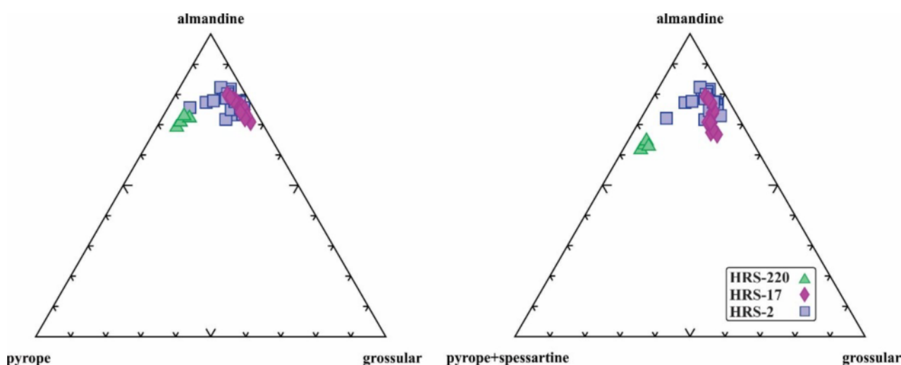
شکل ۶ موقعیت گارنت‌ها در نمودارهای مثلثی \text{Al-Sp+Py-Gr} و \text{Al-Py-Gr} [۲۴]، که براساس آنها ترکیب غالب گارنت‌ها آلماندین است.
