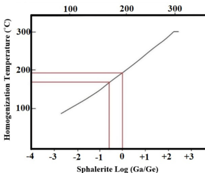
شکل ۶ نمودار دمای همگن‌شدگی نسبت به لگاریتم Ga/Ge برای اسفالریت‌های معدن انگوران که نشان‌دهنده دمای 170^{\circ}\text{C} - 190^{\circ}\text{C} است. بر گرفته از مراجع [۲۲، ۲۱].
