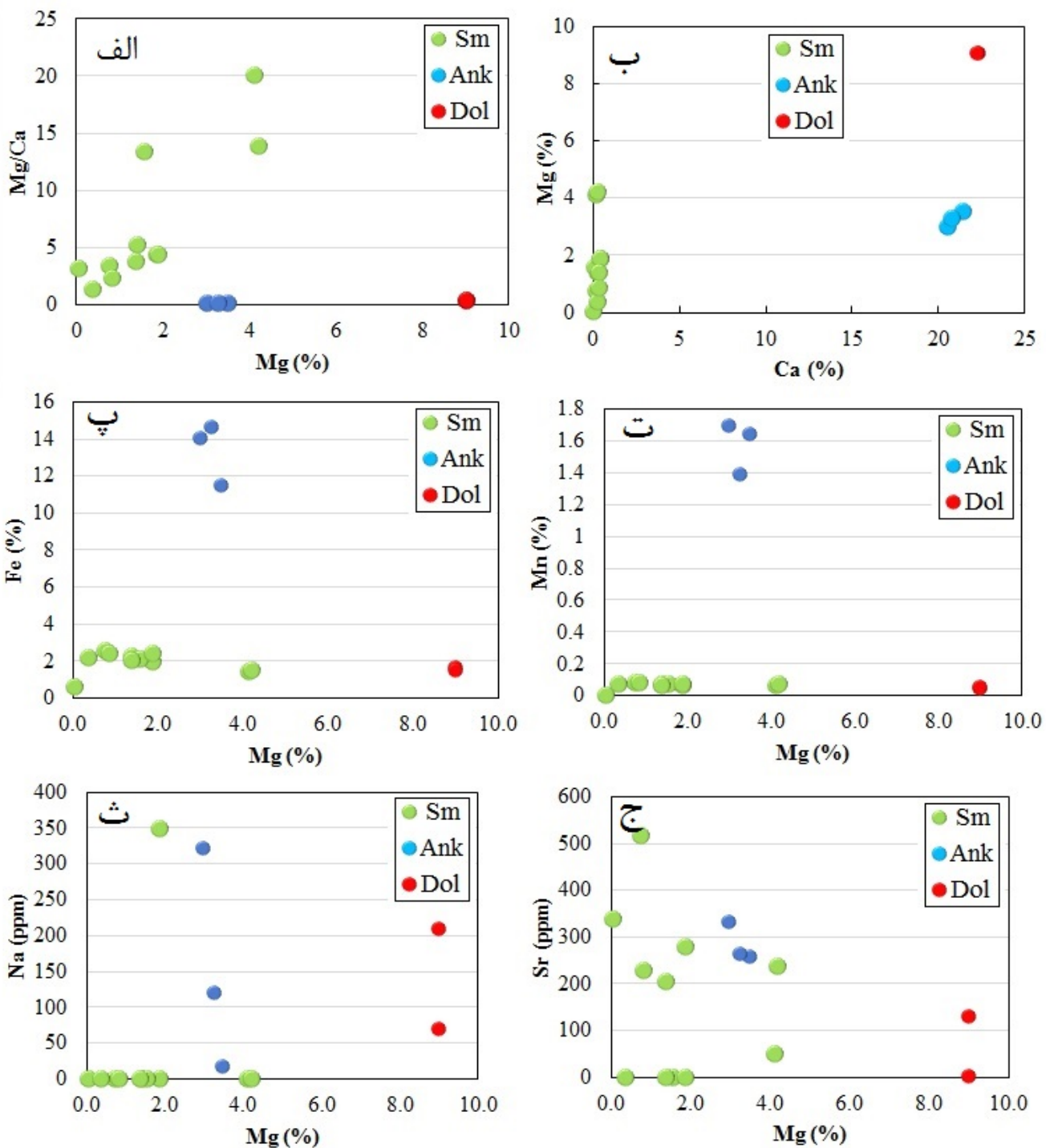
شکل ۴ نمودارهای الف: تغییرات Mg/Ca نسبت به Mg در کربنات‌های معدن انگوران، ب: تغییرات Mg نسبت به Ca، پ: تغییرات Fe نسبت به Mg، ت: تغییرات Mn نسبت به Mg، ش: تغییرات Na نسبت به Mg و ج: تغییرات Sr نسبت به Mg در کربنات‌های معدن انگوران. (Dol: دولومیت، Ank: آنکريت، Sm: اسمیت‌زونیت [۱۵]).
