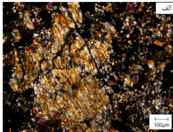
شکل ۹ الف- تصویر میکروسکوپی و ب- تصویر الکترونی پس پراکنده (BSE) از نمونه پیروکسن تجزیه شده (نمونه N.B.C.169-C4)
