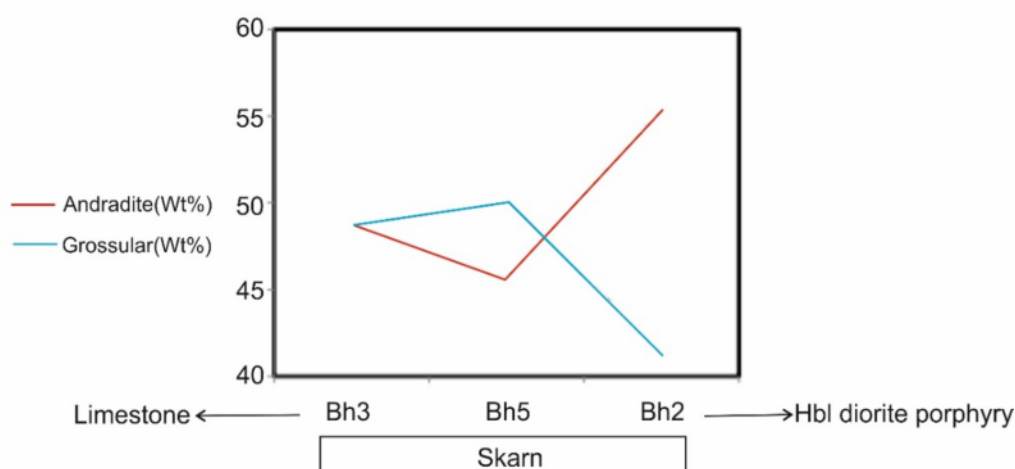
شکل ۶ میانگین تغییرات درصد وزنی آن‌درایت و گروسولار از توده نیمه‌عمیق به سمت سنگ آهک.
