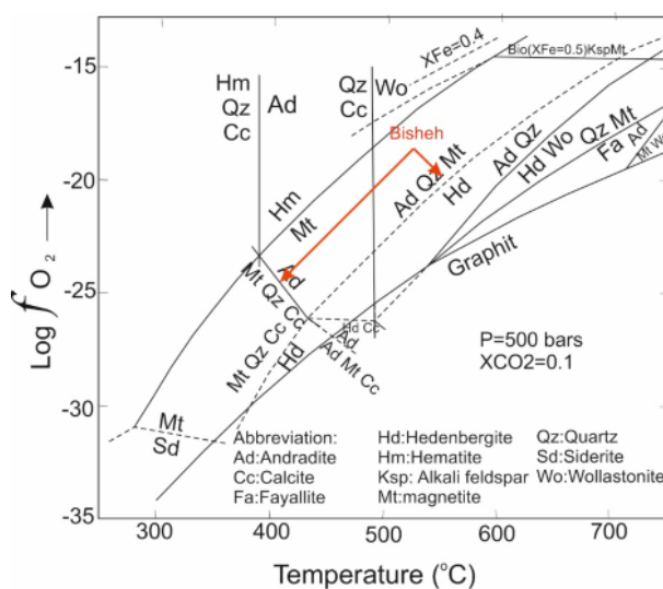
شکل ۱۴ نمودار روابط فازي LOG fO2-T در XCO2=0.1 و فشار ۵۰۰ بار برای سامانه Ca-Fe-Si-C-O-H. [۳۶].
