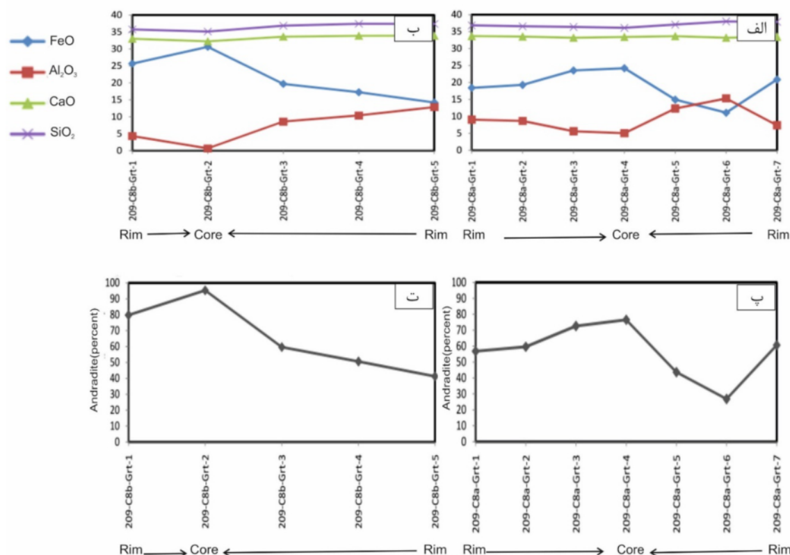
شکل ۸ الف و ب- تغییرات درصد وزنی اکسیدهای \text{FeO} ، \text{Al}_2\text{O}_3 ، \text{CaO} ، \text{SiO}_2 در مرکز و لبه بلورهای گارنت شکل ۵، پ و ت- تغییرات درصد وزنی آندرادیت در بلورهای گارنت شکل ۵ از مرکز به سمت لبه.
