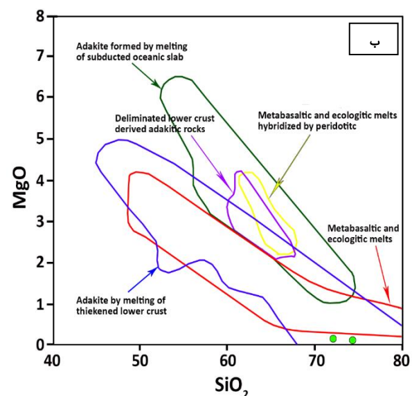
شکل ۱۲ الف) نمودار جداسازی سنگ‌های آداکیتی سیلیس بالا (HSA) و سیلیس پایین (LSA) [۳۹] و ب) و نمودار تعیین خاستگاه سنگ‌های آداکیتی [۴۰] برای نمونه‌های مورد بررسی.
