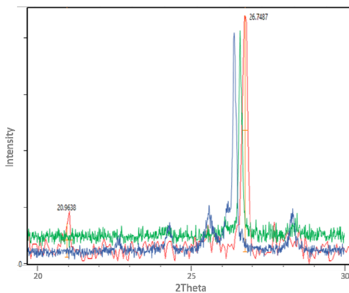
شکل ۷. مقایسه طیف XRD بیوتیت ششگوشی بروجرد (قرمز) با بیوتیت تک میل کانادا (سبز) [۳۵] و آمریکا (آبی) [۳۲].
