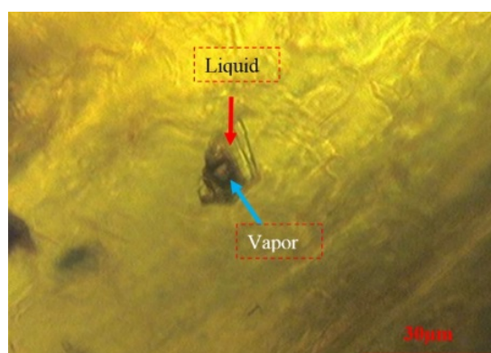
شکل ۱۰ سیال‌های درگیر در کان‌های گارنت نوع آندرادیت. میانبار دو فاز غنی از مایع آبگین و بخار. این میانبارها اولیه بوده و در راستای زوایای خطوط رشد گارنت دیده شده‌اند.
