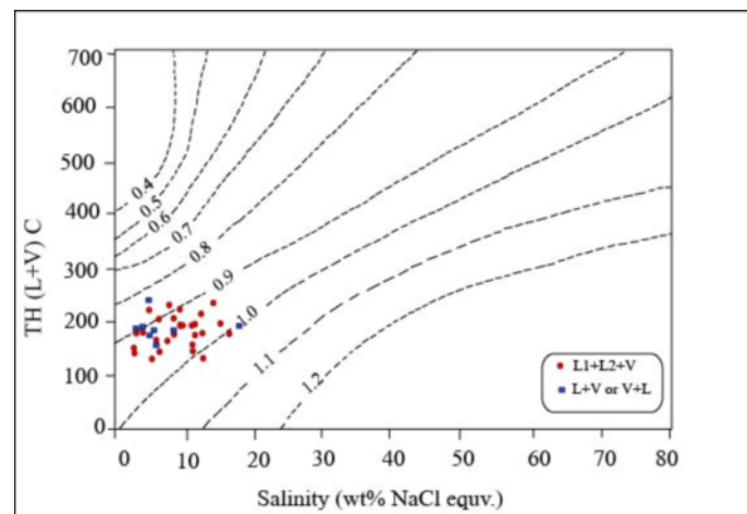
شکل ۸. نمودار دوتایی دمای همگن- شوری [۱۴] برای تعیین چگالی سیال‌های درگیر.
