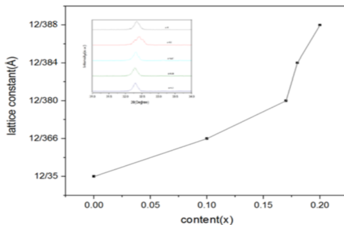
شکل ۲ تغییرات ثابت شبکه نانو ذرات \text{Y}_{2.5}\text{Bi}_{0.5}\text{Fe}_{2-2x}\text{Sn}_x\text{Fe}_{3-x}\text{V}_x\text{O}_{12} با مقدار جانسانی (x).
