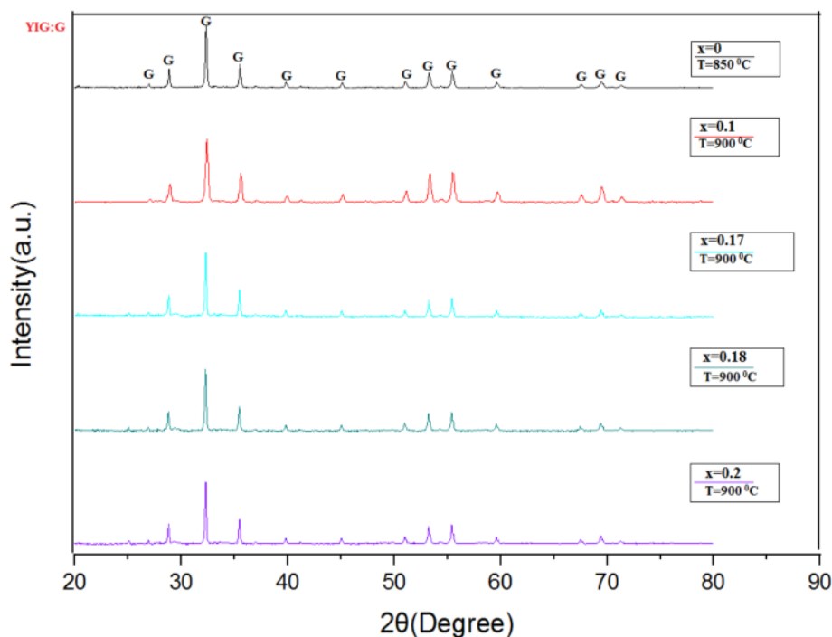
شکل ۱ الگوهای پراش پرتو ایکس نمونه‌های \text{Y}_{2.5}\text{Bi}_{0.5}\text{Fe}_{2-2x}\text{Sn}_x\text{Fe}_{3-x}\text{V}_x\text{O}_{12} با مقادیر جانسانی x = 0.0, 0.1, 0.17, 0.18, 0.2
