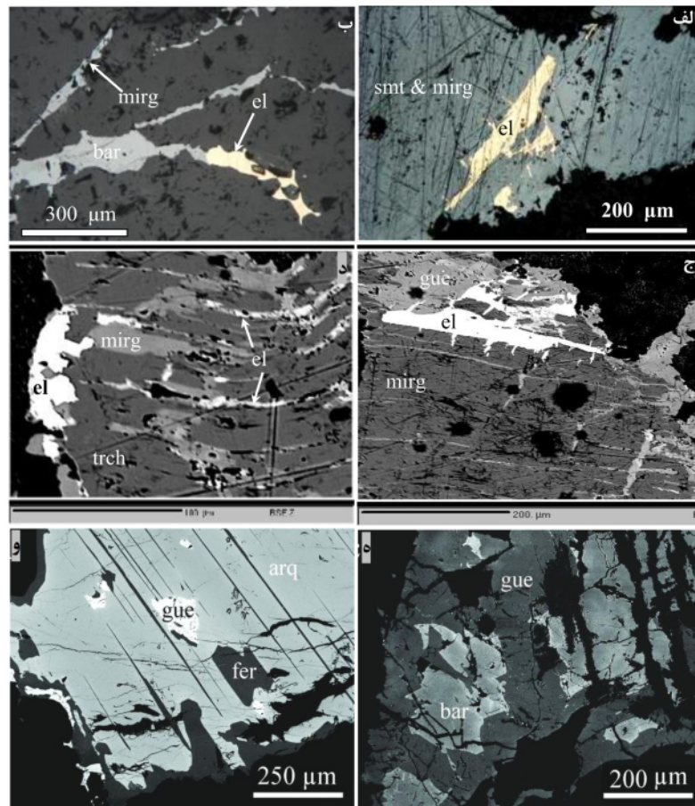
شکل ۶ تصاویر میکروسکوپ نوری بازتابی (الف، ب، ث، ج) و تصاویر میکروسکوپ الکترونی (BSE) (پ و ت) از رخداد برخی سولفوسالت‌ها و الکتروم در کانسنگ‌های طلادار باریکا: (الف) الکتروم در همراهی با اسمایتیت و میرارژیریت، (ب) الکتروم در همراهی با باریکائیت و میرارژیریت، (پ) الکتروم در همراهی با گتاردیت و میرارژیریت، (ت) الکتروم در همراهی با میرارژیریت و تریچمانیت، (ث) باریکائیت، به‌طور قابل توجهی توسط گتاردیت جانشین شده است. (ج) گتاردیت و فردوسی‌ایت به‌طور قابل توجهی توسط آرسن‌کواتراندوریت جانشین شده‌اند. (ارق) آرسن‌کواتراندوریت، bar: باریکائیت، el: الکتروم، fer: فردوسی‌ایت، mirg: میرارژیریت، smit: اسمایتیت، trch: تریچمانیت و gue: گتاردیت).
