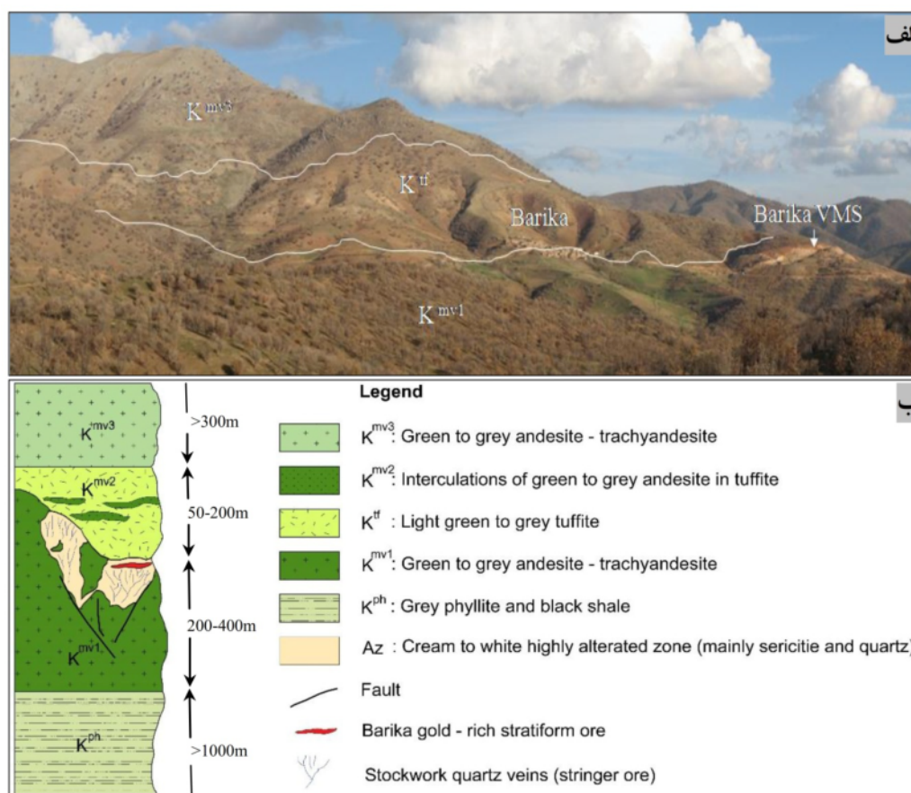
شکل ۲ (الف) نمائی از توالی واحدهای سنگی در منطقه معدنی باریکا. کانسار باریکا در واحد گدازه‌ای ( K^{mv1} ) و در زیر واحد توفیتی ( K^{tf} ) قرار دارد. (ب) توالی چینه‌ای سنگ‌های کرتاسه در منطقه باریکا [۱۵].
