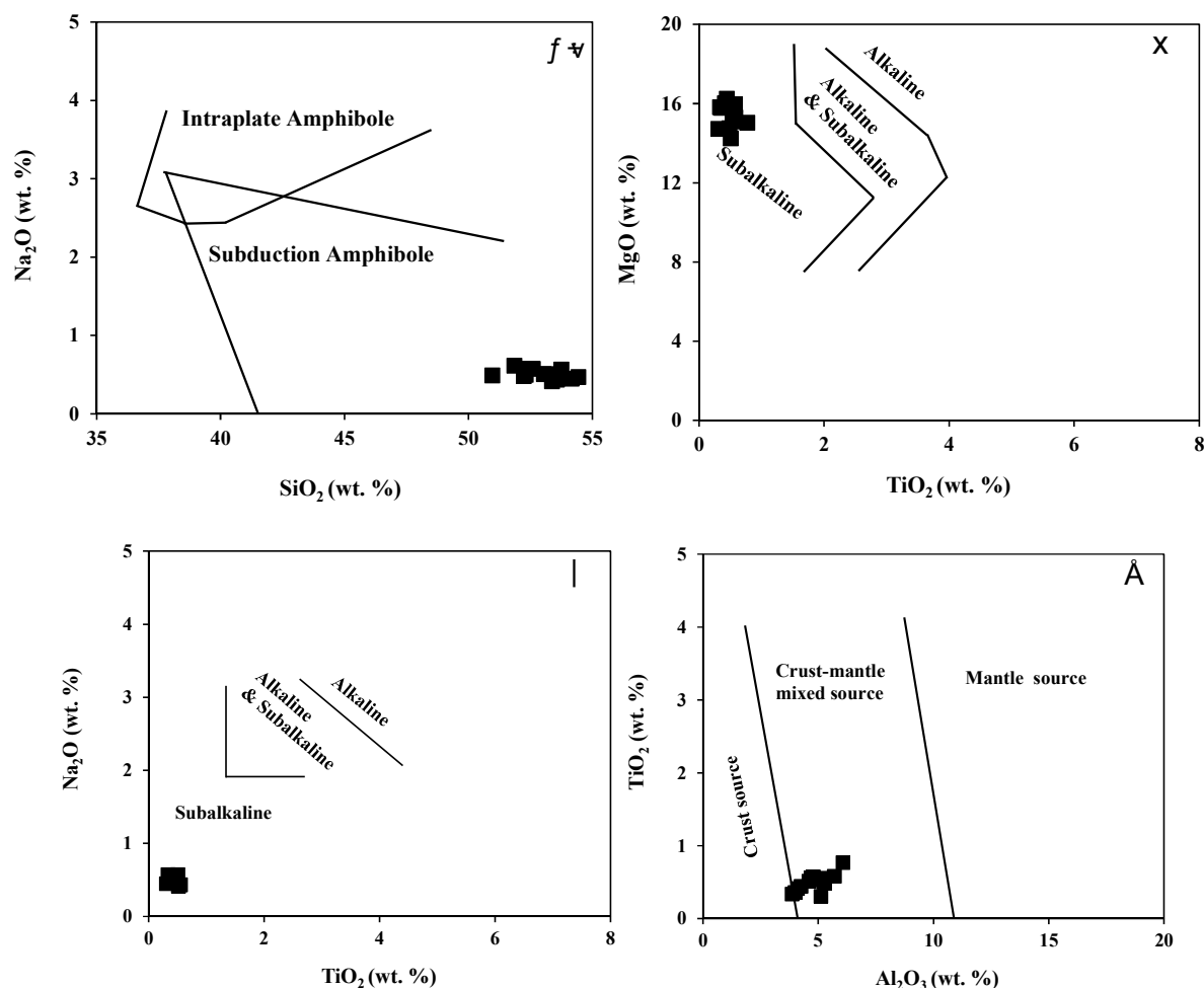
شکل ۴ الف) نمودار \text{Na}_2\text{O} نسبت به \text{SiO}_2 [۲۹] که نشان دهنده ارتباط آمفیبول‌های مورد بررسی با محیط زمین‌ساختی فروانشی است. ب و پ) تعیین ماهیت پلاژیوگرانیت‌های دهسرد با استفاده از ترکیب شیمی آمفیبول‌ها [۳۰]. ت) نمودار \text{TiO}_2 - \text{Al}_2\text{O}_3 که نشان‌دهنده ترکیب ماگمای گوشته‌ای با مواد پوسته‌ای در تشکیل هورنبلندهاست [۳۱].
