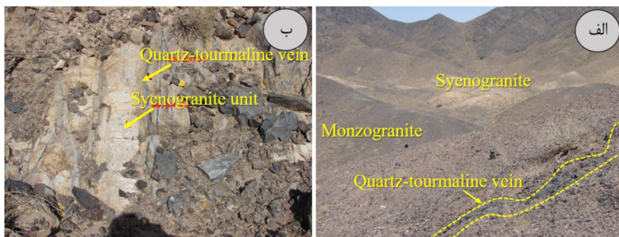
شکل ۳ الف) رخنمون واحد سینوگرانیتی در منطقه شاهکوه، ب) محل برخورد واحد سینوگرانیتی با رگه‌های کوارتز-تورمالین.
