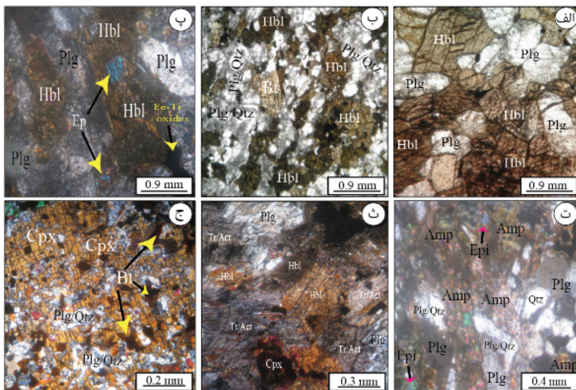
شکل ۳ مقاطع میکروسکوپی متابازیت‌ها (آمفیبولیت‌ها): (الف) آمفیبولیت‌های معمولی (در نور قطبیده صفحه‌ای، PPL)، (ب) بیوتیت آمفیبولیت‌ها (نور PPL)، (پ) اپیدوت آمفیبولیت‌ها (در نور قطبیده مقاطع XPL)، (ت) بیوتیت - اپیدوت آمفیبولیت‌ها (نور XPL)، (ث) ترمولیت - اکتینولیت آمفیبولیت‌ها (نور XPL) و (ج) بیوتیت - کلینوپروکسن آمفیبولیت (نور PPL). نشانه‌های اختصاری کانی‌ها برگرفته از مرجع [۹].
