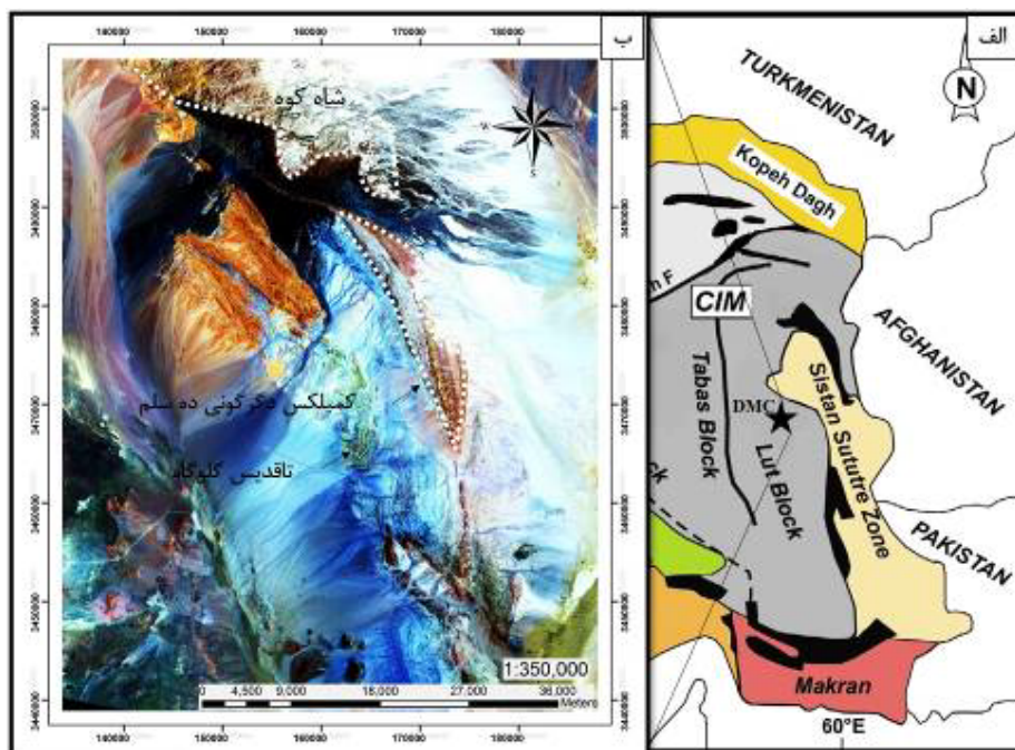
شکل ۱ الف) موقعیت مجموعه دگرگونی دهسلم در کرانه شرقی خرد قاره ایران مرکزی و قطعه لوت [۲۶]: ب) تصویر ماهواره‌ای مجموعه دگرگونی دهسلم و موقعیت آن در جنوب گرانتیت شاه‌کوه (برگرفته از تصاویر ماهواره‌ای لندست).
