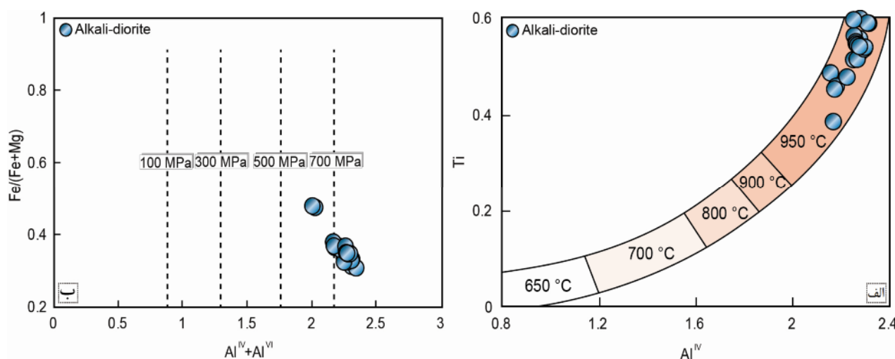
شکل ۹ الف- نمودار Ti نسبت به Al IV برای تعیین دمای تبلور آمفیبول‌های کلسیمی در دیوریت‌های قلیایی [۴۲] و ب- نمودار تغییرات Fe/(Fe+Mg) نسبت به Al IV +Al VI برای تعیین فشار تبلور احتمالی آمفیبول‌ها [۴۴].
