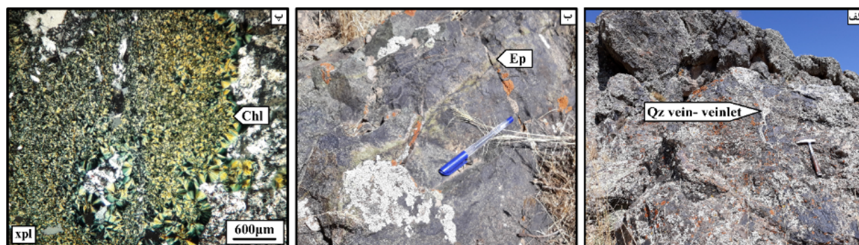
شکل ۳ تصاویر صحرایی و میکروسکوپی از پهنه‌های دگرسانی در منطقه قره‌چای: (الف) برونزد صحرایی از دگرسانی سیلیسی، (ب) نمای از رگچه‌های اپیدوتی موجود در واحد آندزیتی در رخنمون صحرایی و (پ) کلریت‌های سبز رنگ با بافت شعاعی که پیامد دگرسانی کانی‌های فرومنیزین موجود در واحد آندزیتی هستند. نام اختصاری کانی‌ها برگرفته از مرجع [۹] است. (Qz: کوارتز، Ep: اپیدوت و Chl: کلریت).
