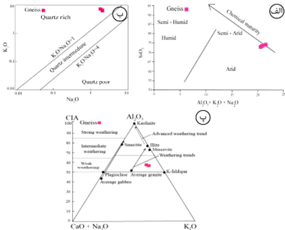
شکل ۷ الف) نمودار دوتایی \text{SiO}_2 نسبت به \text{Al}_2\text{O}_3 + \text{K}_2\text{O} + \text{Na}_2\text{O} [۲۷] برای بررسی وضعیت دیرینه اقلیم سنگ مادر گنیس‌های منطقه مورد بررسی، ب) نمودار \text{K}_2\text{O} نسبت به \text{Na}_2\text{O} [۲۸] برای تعیین مقدار کوارتز در رسوب‌های سنگ خاستگاه گنیس‌ها و پ) نمودار \text{ACNK} [۲۹] برای تعیین درجه هوازدگی سنگ آذرین خاستگاه رسوب‌های گنیس‌های شرق سلماس.
