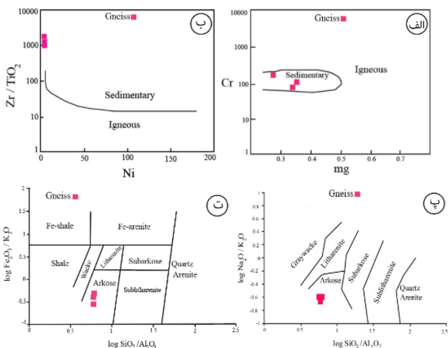
شکل ۶ الف و ب) نمودارهای دوتایی \text{Cr-mg} و \text{Zr/TiO}_2 - \text{Ni} [۱۹]. برای بررسی سنگ مادر رسوبی و آذرین گنیس‌های مجموعه دگرگونی منطقه از نوع رسوبی یا پاراگنیس است. \text{mg} از اعداد نیگلی است، پ و ت) که بر این اساس، خاستگاه آنها نمودارهای دوتایی بر پایه تغییرات لکارتیمی \text{Na}_2\text{O/K}_2\text{O} و \text{Fe}_2\text{O}_3/\text{K}_2\text{O} نسبت به \text{SiO}_2/\text{Al}_2\text{O}_3 [۲۰] برای تعیین نوع سنگ رسوبی مادر گنیس‌های منطقه که بر این اساس بیشتر از نوع آرکوز است.
