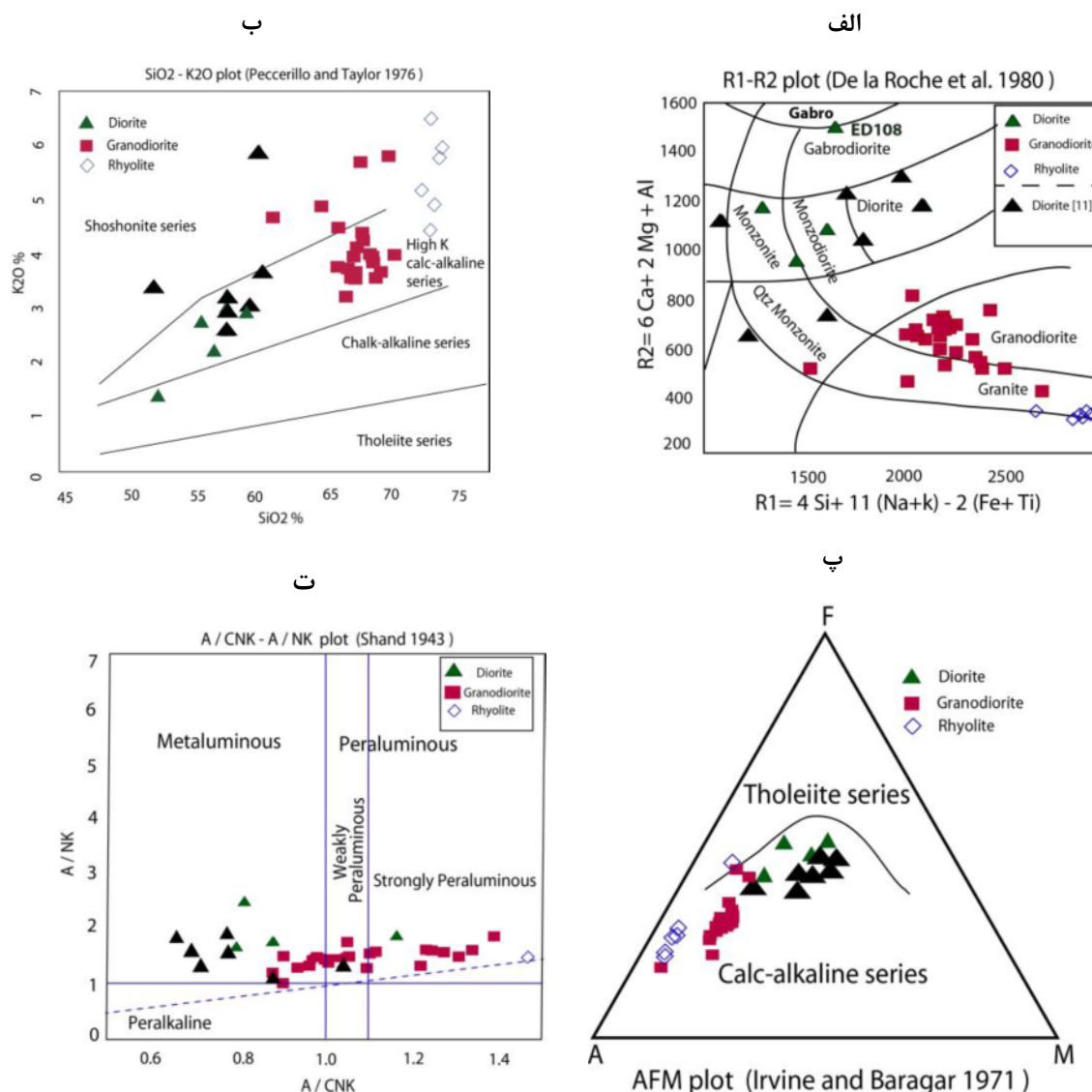
شکل ۵. جانمایی نمونه‌ها در الف: نمودار R1-R2 [۱۸] که باساز آن، نمونه ED108 مافیکترین و بازیگترین نمونه بوده که میزبان نفوذ توده گرانودیوریتی است. ب: نمودار K_2O نسبت به SiO_2 که نشان دهنده ماهیت کلسیمی-قلیایی غنی از پتاسیم نمونه‌هاست [۲۰]. پ: نمودار AFM [۲۱] که نشان دهنده کلسیمی-قلیایی بودن همه نمونه‌هاست. ت: نمودار اصلاح شده A/CNK-A/NK [۲۲] که نشان می‌دهد که همه نمونه‌های ریولیتی در گستره پرالومین، گرانودیوریتی متالومین-پرالومین و همه نمونه‌های دیوریتی متالومین هستند. مثلث سبز کوچک نشانگر دیوریت، مثلث‌های سیاه بزرگتر داده‌های دیوریتی مرجع [۱۱]، مربع قرمز گرانودیوریت و لوزی‌های آبی توخالی نمونه‌های ریولیتی هستند.
