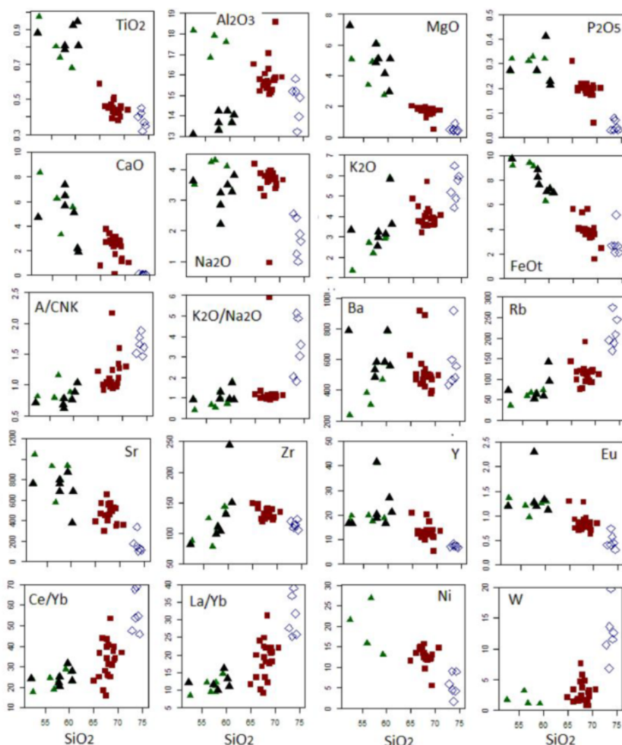
شکل ۶ نمودارهای \text{TiO}_2 , \text{Al}_2\text{O}_3 , \text{MgO} , \text{P}_2\text{O}_5 , \text{CaO} , \text{Na}_2\text{O} , \text{K}_2\text{O} , \text{FeO}_t , A/CNK, \text{K}_2\text{O/Na}_2\text{O} (به درصد) و عناصر فرعی Sr, Rb, Ba, Ni, W, La/Yb, Ce/Yb, Y, Zr (به ppm) نسبت به \text{SiO}_2 . نشانه‌ها شبیه شکل ۵ هستند.
