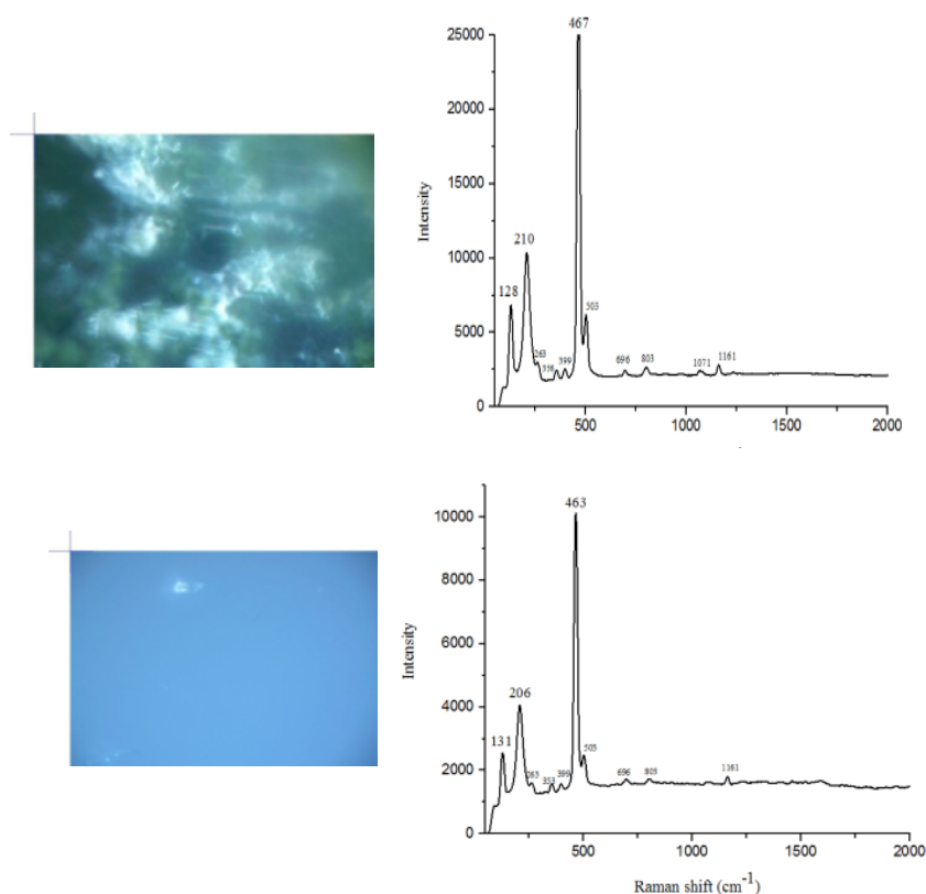
شکل ۱۰ تصویر میکروسکوپی و طیف‌های رامان کوارتز، موگانیت، همتایت و کلسیت در الف) آگات‌های خزهای و ب) آگات تخم مرغی .
