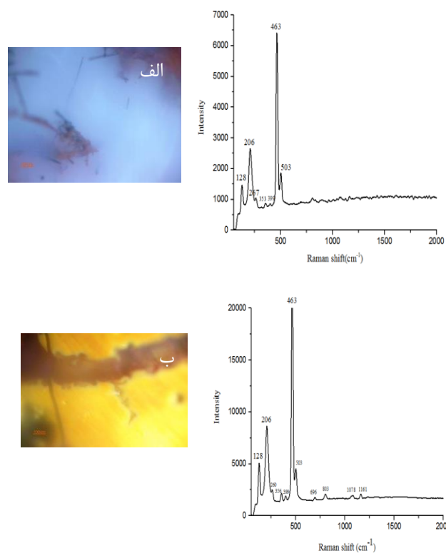
شکل ۱۱ الف. تصاویر میکروسکوپی و طیف‌های رامان کوارتز، مoganیت و هماتیت در ژاسپرهای شاخه ای الف) خاکستری و ب. زردرنگ
