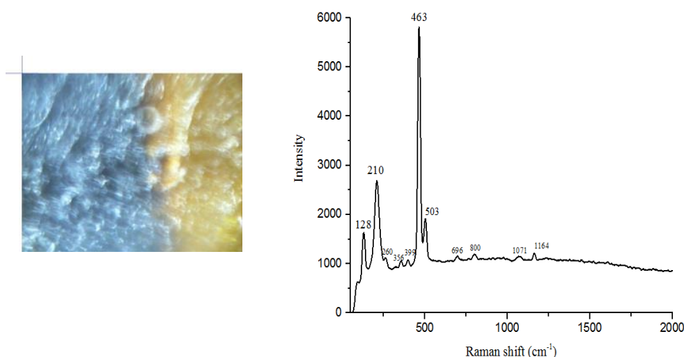
شکل ۱۲ تصویر میکروسکوپی و طیف رامان کوارتز، موگانیت، هماتیت و کلسیت در ژاسپرهای نواری.
