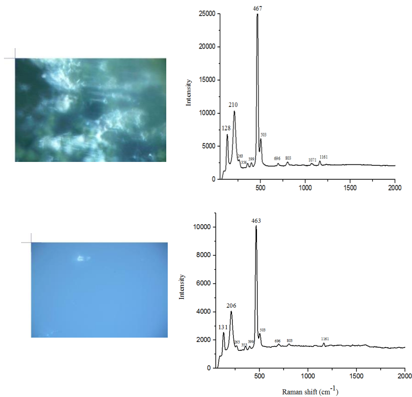
شکل ۱۰ تصویر میکروسکوپی و طیف‌های رامان کوارتز، مoganیت، هماتیت و کلسیت در الف) آگات‌های خزه‌ای و ب) آگات تخم مرغی.
