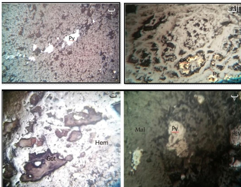
شکل ۱۰ مقطع صیقلی الف) کالکوپیریت و پیریت، ب) پیریت، پ: پیریت، هماتیت و مالاگیت و ت) هماتیت و گوتیت
