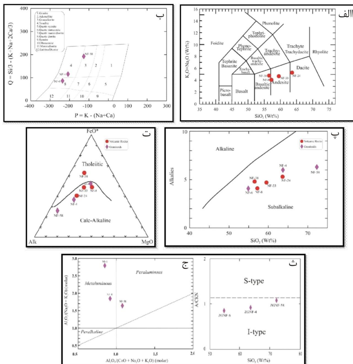
شکل ۶ الف) نمودار مجموع قلیایی نسبت به سیلیس (TAS)، ب) نمودار نامگذاری شیمیایی سنگ‌های درونی [۱۳]، پ) نمودار \text{SiO}_2 نسبت به (\text{Na}_2\text{O}+\text{K}_2\text{O}) [۱۴]، ت) نمودار جدا کننده سری تولیتی از سری آهکی قلیایی، ث) نمودار پیشنهادی [۱۵]، ج) نمودار [۱۶] که براساس آن گرانیتوئید های منطقه در گستره I قرار دارند.
