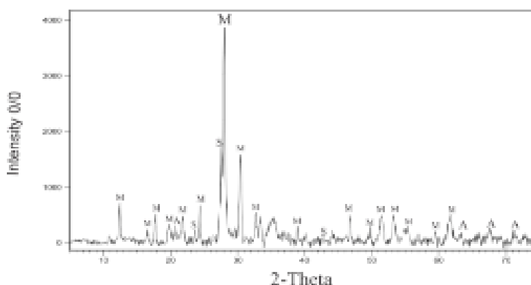
شکل ۶ الگوی XRD نمونه‌ی TP1 سنتز شده در حضور LiOH با غلظت ۰٫۲۵ مول بر لیتر، در دمای ۱۵۰ درجه‌ی سانتی‌گراد برای ۷۲ ساعت. (M: مرلینوئیت، S: سانیدین و A: آلبیت).
