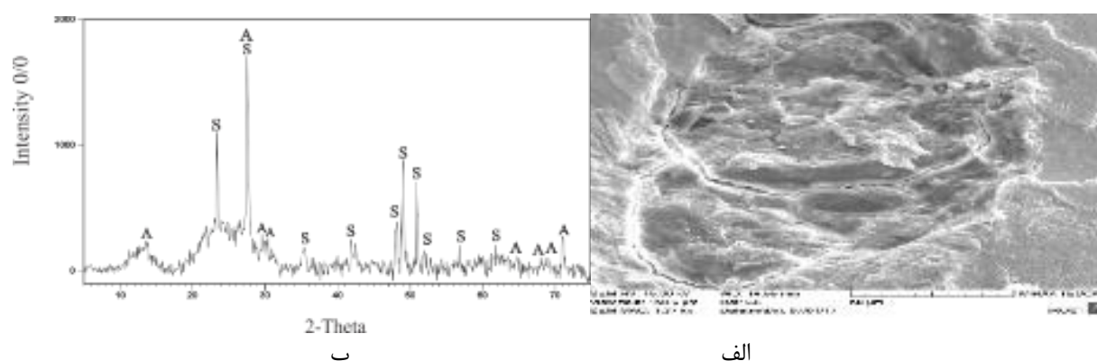
شکل ۵ الف) الگوی پراش پرتو ایکس (XRD) نمونه‌ی اولیه پرلیت؛ S نشانگر کانی سانیدین و A نشانگر کانی آلبیت است. ب) تصویر SEM از نمونه‌ی اولیه (پرلیت).
