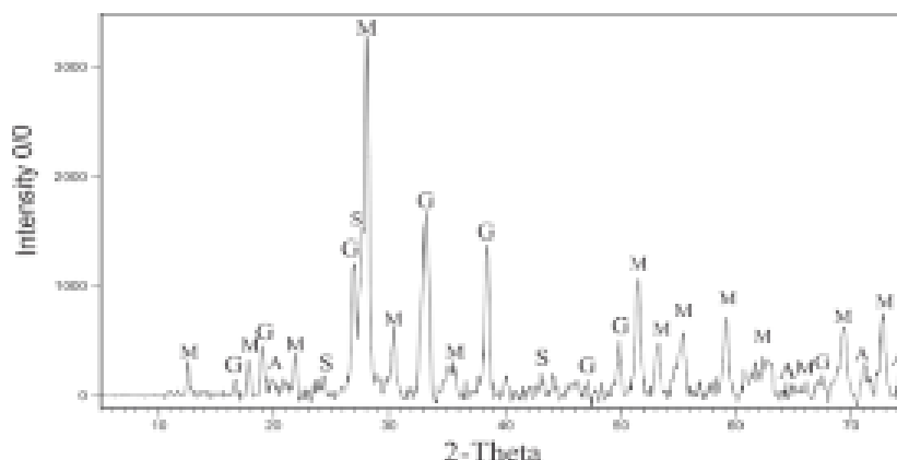
شکل ۸ الگوی XRD نمونه‌ی TP2 سنتز شده در حضور LiOH با غلظت ۰/۵ مول بر لیتر در دمای ۱۵۰ درجه سانتی گراد برای ۷۲ ساعت. (G: ژیسمونندین، M: مرلینوئیت، S: سانیدین، A: آلبیت).
