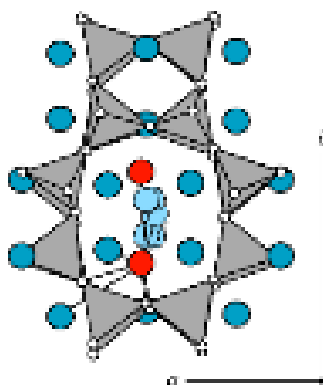
شکل ۴ مدل هم آرای کانی ژیسمونندین. علائم آبی پررنگ: ملکول آب آزاد، قرمز: کاتیون کلسیم و آبی روشن: ملکول آب پیوندی را نشان می‌دهند [۲۵].
