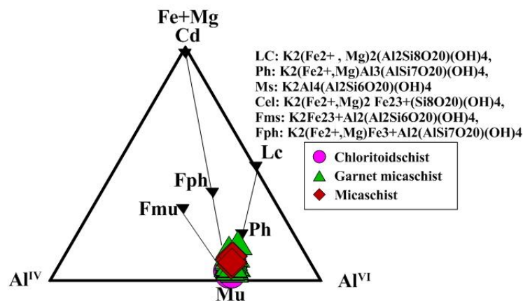
شکل ۶. نمودار تعیین ترکیب مسکوویت‌ها [۲۵] که مسکوویت‌های مورد بررسی بین قطب‌های مسکوویت و فنزیت قرار دارند.
