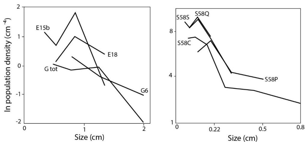
شکل ۹ نمودارهای توزیع ابعاد بلورهای گارنت موجود در الف) هورنفلس‌های دوره اشنویه و ب) شیست‌های شاهیندر (SMC).
