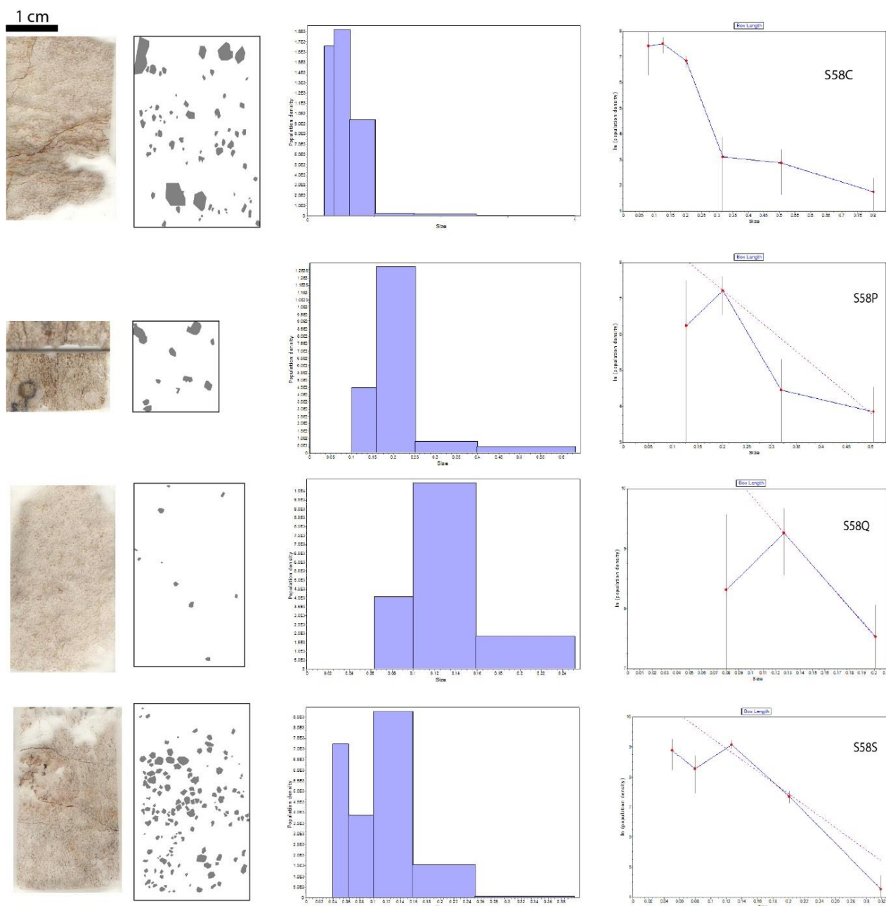
شکل ۸ طرحواره مقاطع نازک از شکفته بلورهای گارنت، نمودار تجمعی ستونی برای دانه‌های گارنت و نیز نمودار توزیع ابعاد بلوری برای گارنت‌های موجود در شایست‌های شاهیندژ (SMC).
