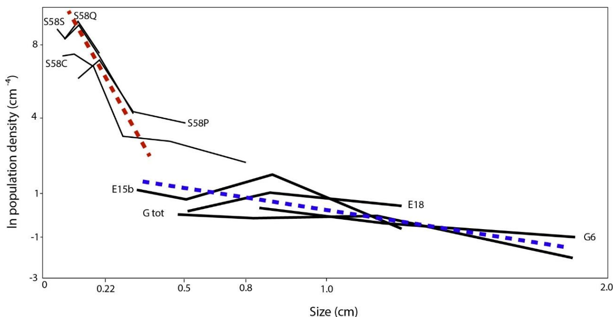
شکل ۱۰ مقایسه الگوی CSD گارنت‌های شیست‌های شاهیندر (خطوط سیاه نازک) با هورنفلس‌های دوره (خطوط سیاه پر رنگ). شیب خط وایزش چشمی برای شیست‌های شاهیندر با خط چین قرمز و برای هورنفلس‌های دوره با خط چین آبی نشان داده شده است.
