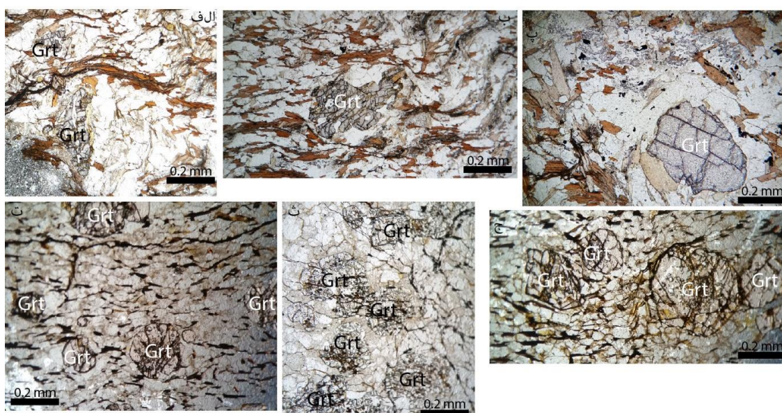
شکل ۵ تصاویر میکروسکوپی از شلیست‌های گارنت‌دار شاهیندژ (SMC) بصورت منفرد در متن جهت‌یافته سنگ.
