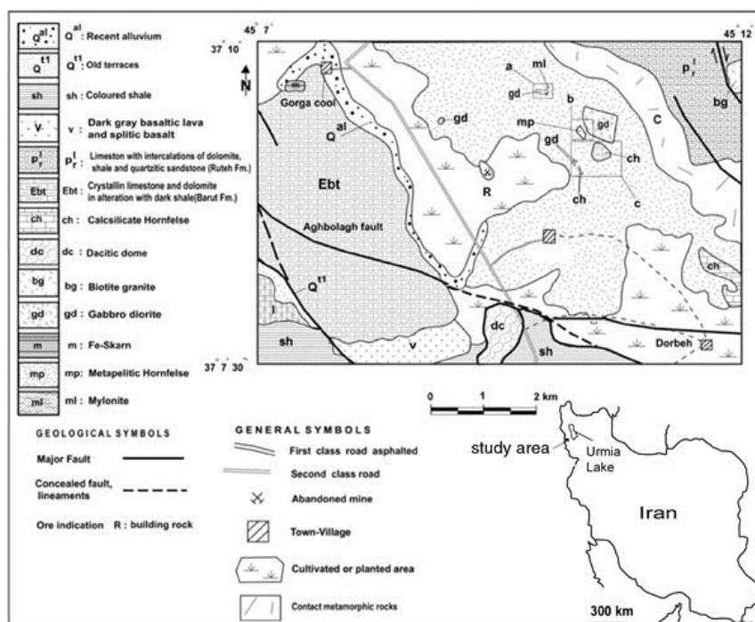
شکل ۲ نقشه زمین‌شناسی ساده شده از توده نفوذی اسلاملو و هاله مجاورتی منطقه دوربه اشویه در جنوب آذربایجان غربی [۳۲].
