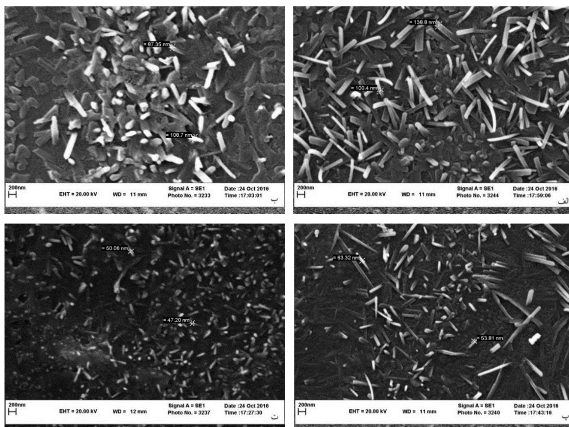
شکل ۳ تصاویر SEM لایه‌های پنتاکسید واندیوم (الف) خالص، (ب) با ۱۰، (پ) ۲۰ و (ت) ۳۰ درصد وزنی ایندیوم.
