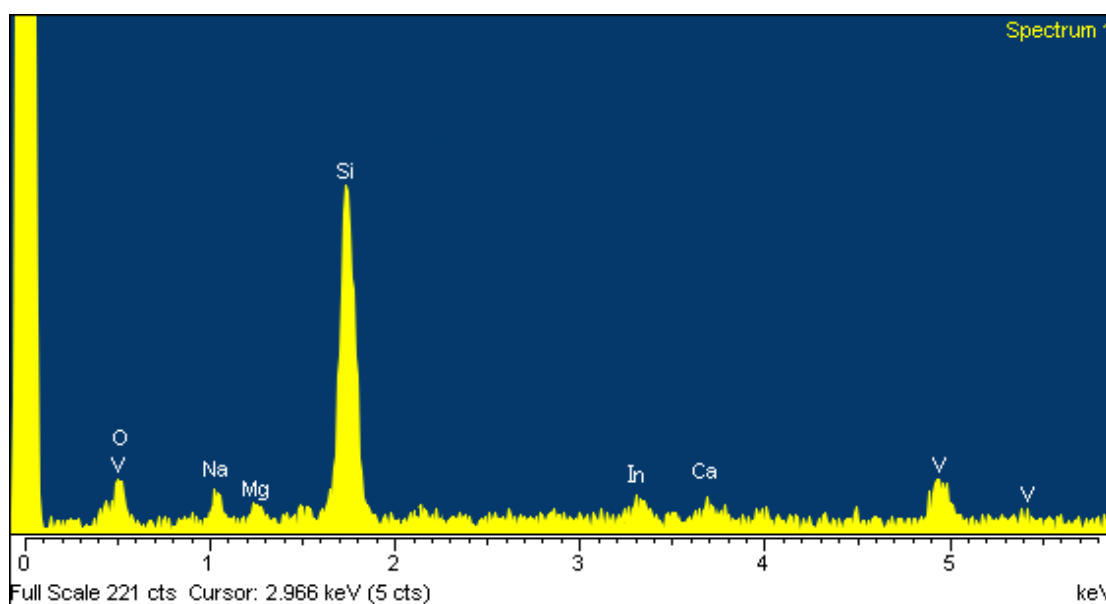
شکل ۴ طیف EDX لایه پنتاکسید وانادیوم با ۳۰ درصد وزنی ایندیوم در محلول.
