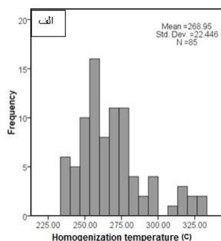
شکل ۷ نمودارهای ستونی مربوط به سیال‌های درگیر: الف) دمای همگن‌شدگی و ب) مقدار شوری.
