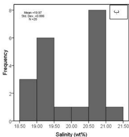
شکل ۷ نمودارهای ستونی مربوط به سیال‌های درگیر: الف) دمای همگن‌شدگی و ب) مقدار شوری.
