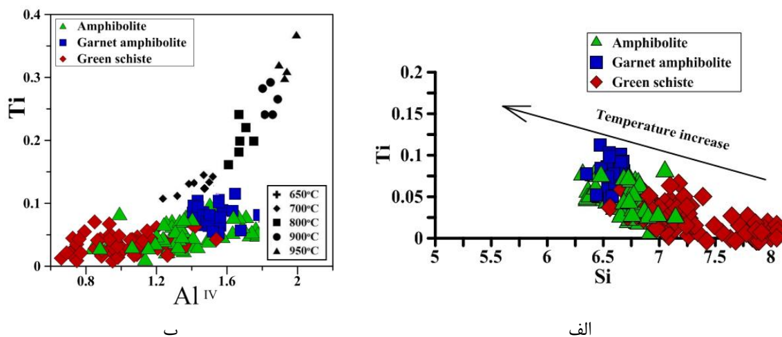
شکل ۸ موقعیت ترکیبی آمفیبول‌های متابازیت‌های مجموعه دگرگونی- آذرین جنوب دو چاه در الف - نمودار تغییرات Si نسبت به Ti [۲۴] و ب- نمودار Al^{IV} نسبت به Ti [۲۵]. که روند افزایش دمای دگرگونی از شیبست سبز به آمفیبولیت در آن به طور کامل نمایان است.
