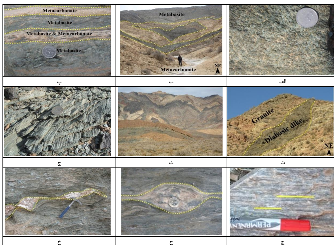
شکل ۳ تصاویری از ویژگی‌های بارز متابازیت‌های مجموعه دگرگونی-آذرین جنوب دوجاه: الف- ساخت بادامکی برجامانده از سنگ مادر بازالتی در متابازیت‌ها. ب و پ- همراهی متابازیت‌ها با کربنات‌ها و وجود میان‌لایه‌های کربناتی در بین آنها که نشانگر تشکیل بازالت‌های مادر در محیط آبی است، ت- دایک دیابازی قطع‌کننده بیوتیت گرانیت‌ها (دید به سمت شمال شرق)، ث- چین‌های با مقیاس ماکروسکوپی در آمفیبولیت‌ها (دید به سمت شمال)، ج- چین‌های موزسکوپی در شیست‌های سبز، چ و خ- به ترتیب خطوارگی مشخص، عدسی‌های سیلیسی به شکل سیگما و بودین‌شدگی رگه‌های سیلیسی موجود در آمفیبولیت که نشان‌دهنده قرارگیری متابازیت‌ها در پهنه‌های برشی هستند.
