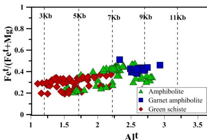
شکل ۹ نمودار Fe/(Fe+Mg) نسبت به Al^I [۲۶] که فشار تشکیل متابازیت‌های مجموعه دگرگونی دو چاه را نشان می‌دهد.
