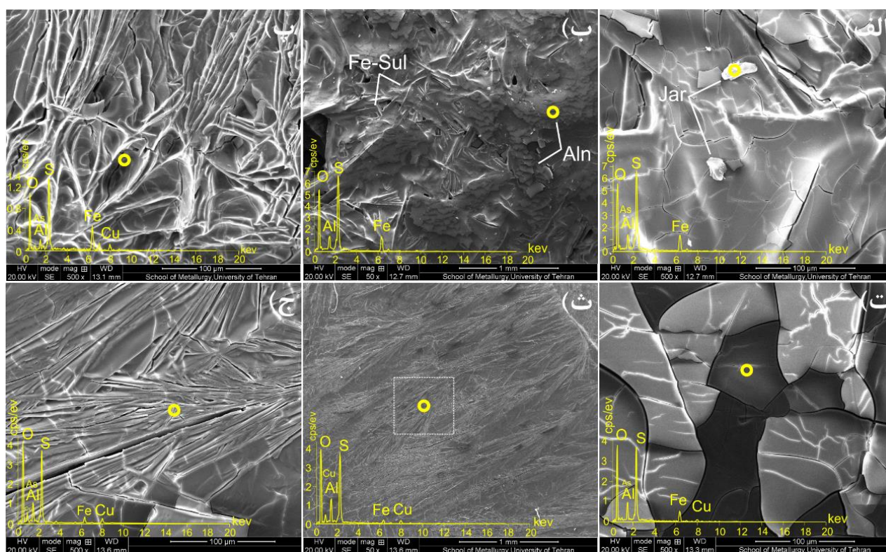
شکل ۴ تصاویر میکروسکوپ الکترونی و تجزیه شیمیایی نقطه‌ای (الف) ژاروسیت (نمونه HC1S)، (ب) آلونژن (Aln) و سولفات آهن (Fe-Sul)، (پ) کوکونیمبیت، (ت) فری کوپاپیت، (ث) سولفات‌های آلومینیم و مس. گستره مشخص شده در تصویر ج آورده شده است، (ج) آنتلریت.
