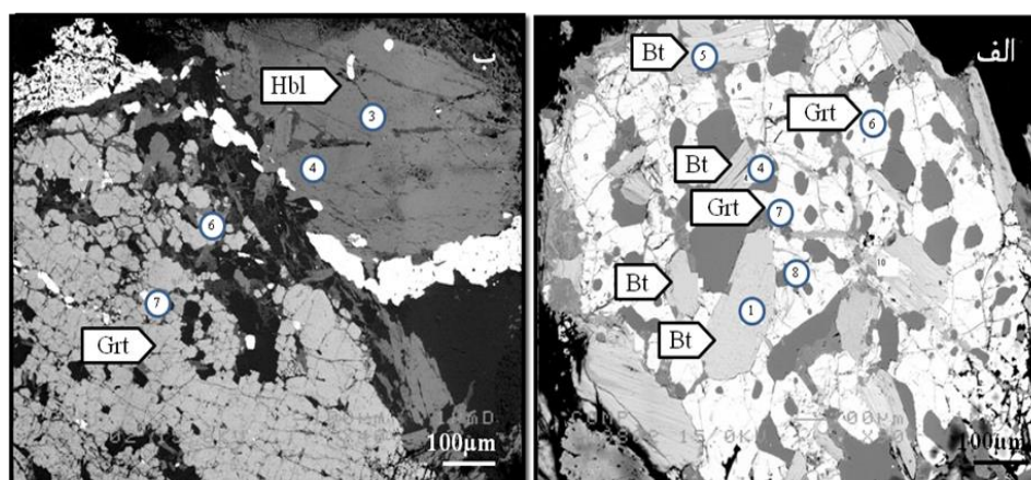
شکل ۶ نقاط تجزیه شده توسط تجزیه ریزکاوا الکترونی که نشان دهنده الف) وجود بیوتیت درون گارنت‌های متاپلیت‌ها و ب) همجواری هورنبلند و گارنت در گارنت آمفیبولیت‌های منطقه گل‌گهر هستند.
