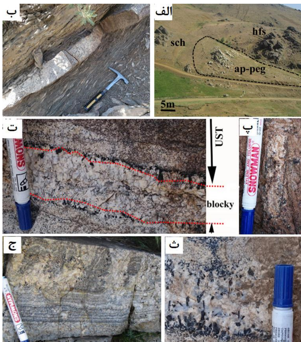
شکل ۲ تصاویر صحرایی منطقه سیمین: الف) تنوع واحدهای سنگی در منطقه سیمین شامل میگماتیت و دایک‌های آپلیت-پگماتیتی، ب) شواهد پهنه برشی در منطقه (اندالوزیت‌های موجود در شیب‌های لبه حالت سیکمونیدی (S شکل) نشان می‌دهند، پ) انباشت تورمالین در لبه آندالوزیت‌های سیلیمانیته شده، ت) ساخت‌های انجماد تک جهته از لبه به سمت مرکز (UST) و ساخت توده‌ای (blocky) در مرکز دایک‌های موجود در منطقه، ث) رشد تورمالین‌ها بصورت عمود بر دیواره در لبه آپلیت-پگماتیت‌ها، ج) ساخت آپلیت نواری در لبه آپلیت-پگماتیت‌ها. آپلیت-پگماتیت=ap-peg، هورنفلس=hfs، شیبست=Sch.
