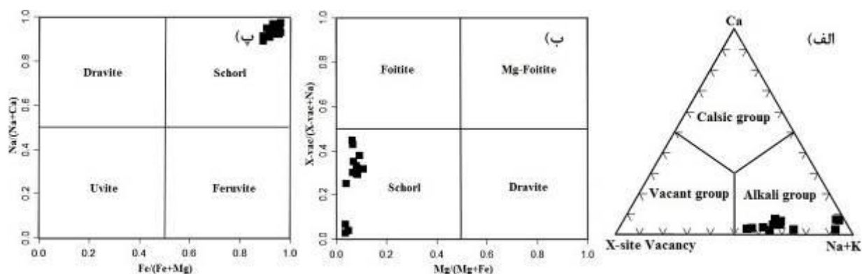
شکل ۴ الف) نمودار مثلثی Ca-(X-vac)-Na+(K) [۱۶]، و جایگاه نمونه‌های مورد بررسی بر آن، ب) جایگاه تورمالین-های مورد بررسی بر نمودار vac/(X-vac+Na)X نسبت به Mg/(Mg+Fe) [۱۹] و پ) جایگاه تورمالین‌ها بر نمودار Na/(Na+Ca) نسبت به Fe/(Fe+Mg) [۲۰].
