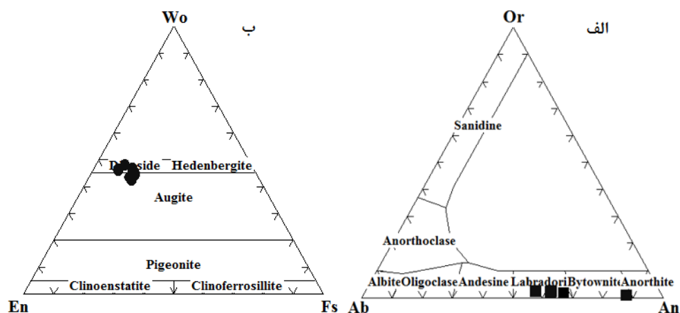
شکل ۴ الف) جایگاه ترکیبی پلاژیوکلازهای موجود در گدازه‌های بازیک مورد بررسی بر نمودار تقسیم‌بندی فلدسپارها [۳۰] و ب) نمودار سه‌تایی En-Wo-Fs [۳۵] برای رده‌بندی کلینوپیروکسن‌ها.
