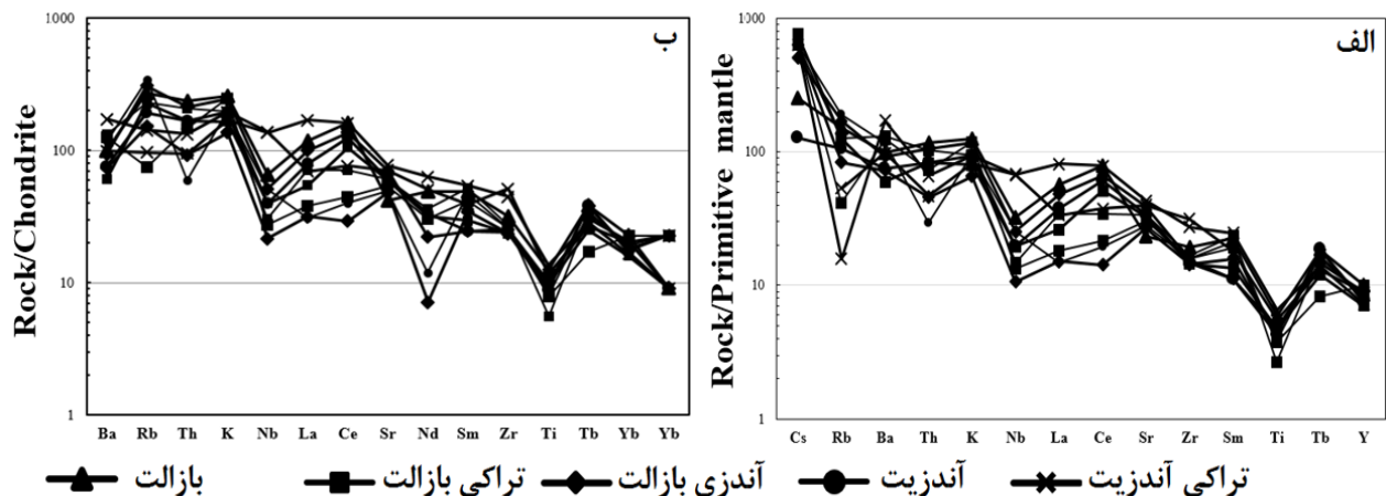
شکل ۷ نمودارهای عنکبوتی (چند عنصری) برای سنگ‌های آتشفشانی مورد بررسی بهنجار شده نسبت به الف ترکیب گوشته اولیه [۴۴]، و ب) کندریت [۴۸]. (بازالت مثلث، آندزیت دایره، تراکی بازالت لوزی، تراکی آندزیت مربع، آندزیت دایره و تراکی آندزیت ضربدر).
