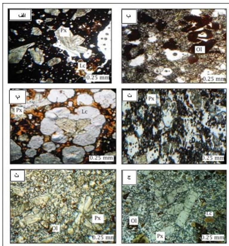
شکل ۳ تصاویر میکروسکوپی از سنگ‌های زیر اشباع از سیلیس مشاهده شده در منطقه در نور PPL. بلورهای لوئیسیتیت، پیروکسن و اولیوین در متن سنگ بصورت درشت بلورهای مشخص حضور دارند. بلورهای پلاژیوکلاز بصورت دانه ریز و ریزسنگی در زمینه‌ای با بافت پورفیری به همراه پیروکسن‌های ریزسنگی حضور دارد. بافت‌های مشاهده شده در سنگ‌ها: (الف) بافت ویتروفیری، (ب) بافت پورفیری، (پ) بافت مشبک، (ت) بافت حفره‌ای، ث: بافت موازی هم‌رشدی، (ج) بافت میان دانه‌ای.
