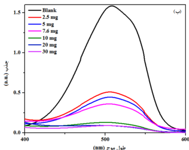
شکل ۱۰ (الف) فرآیند تخریب میتل اورانژ به وسیله BFO-۳ بر حسب زمان تابش خورشید (۲۰ ml محلول ۹ ppm در \text{pH} = ۲ ) و (ب) طیف جذبی UV-Vis نمونه‌ها در پایان زمان اندازه‌گیری.
