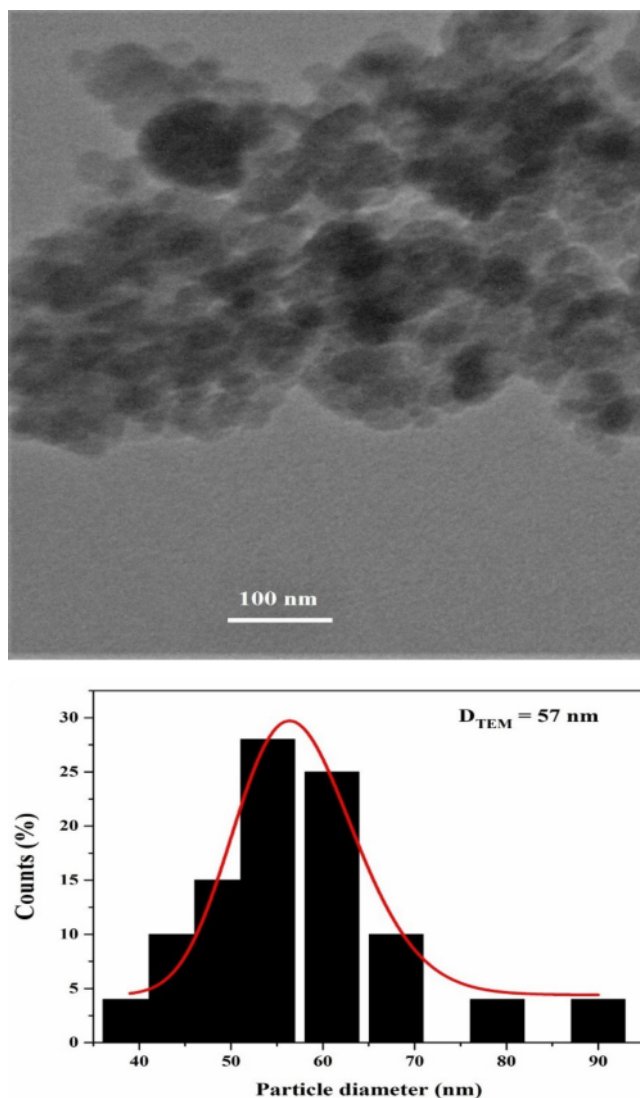
شکل ۶ الف) تصویر TEM و ب) نمودار ستونی توزیع ذرات به همراه برازش آن با تابع توزیع لگاریتم نرمال برای نمونه BFO-3.
