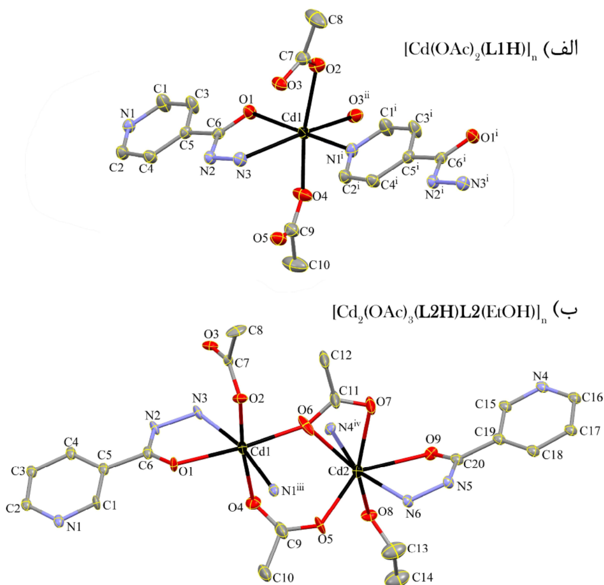
شکل ۲ تصویری از بیضوی گون‌های گرمایی ترکیب‌های الف) [Cd(OAc)_2(L1H)]_n و ب) [Cd_2(OAc)_3(L2H)L2(EtOH)]_n . بیضی‌گون‌های گرمایی با احتمال ۵۰ درصد رسم شده‌اند. به منظور وضوح بیشتر، اتم‌های هیدروژن حذف شده‌اند.
