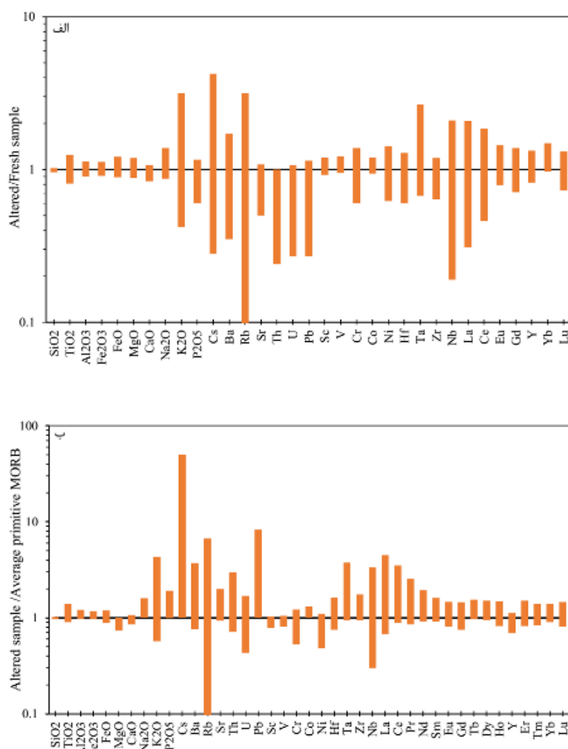
شکل ۶ نمودار بهنجارش نمونه‌ها نسبت به نمونه نسبتاً سالم در منطقه (الف) و نمونه استاندارد (ب).
