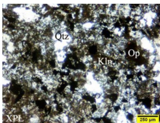
شکل ۹ دگرسانی آرژیلی و تشکیل کانی رسی (Kln).
