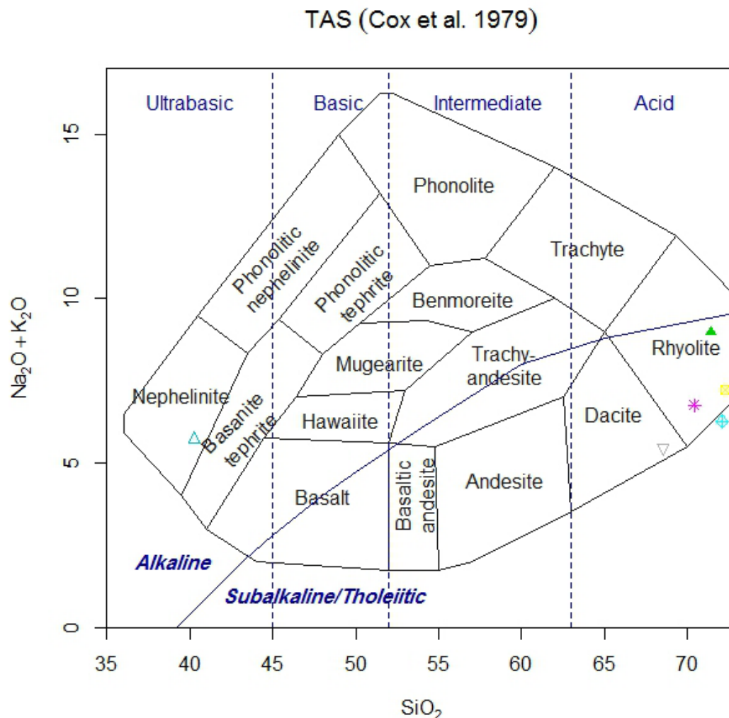
شکل ۱۹ رده بندی سنگ‌های سطحی میزبان آهن و آپاتیت.
