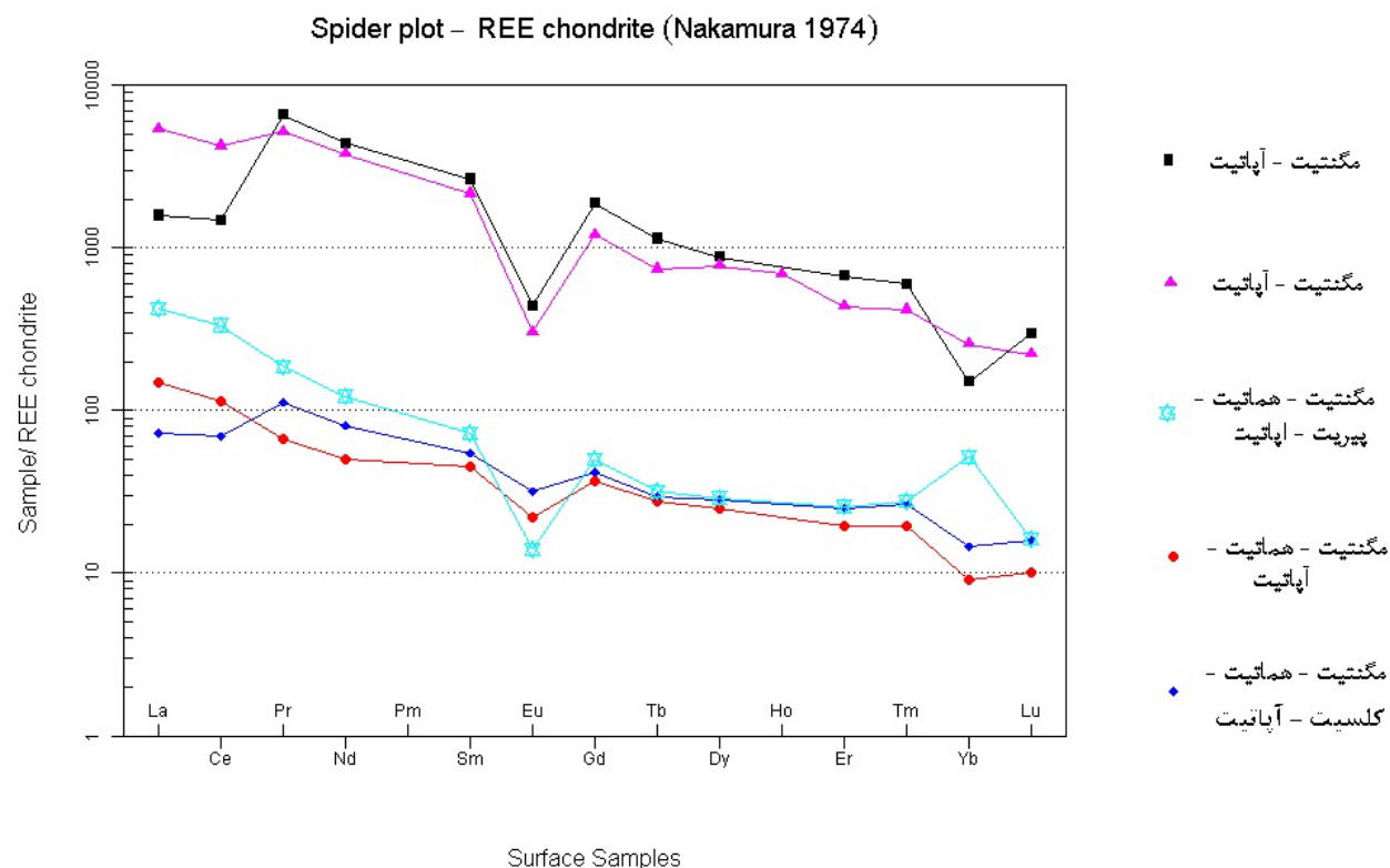
شکل ۱۵ نمودار عنکبوتی عناصر خاکی نادر بر اساس نوع کانی‌سازی و بهنجارش با کاندیت.
