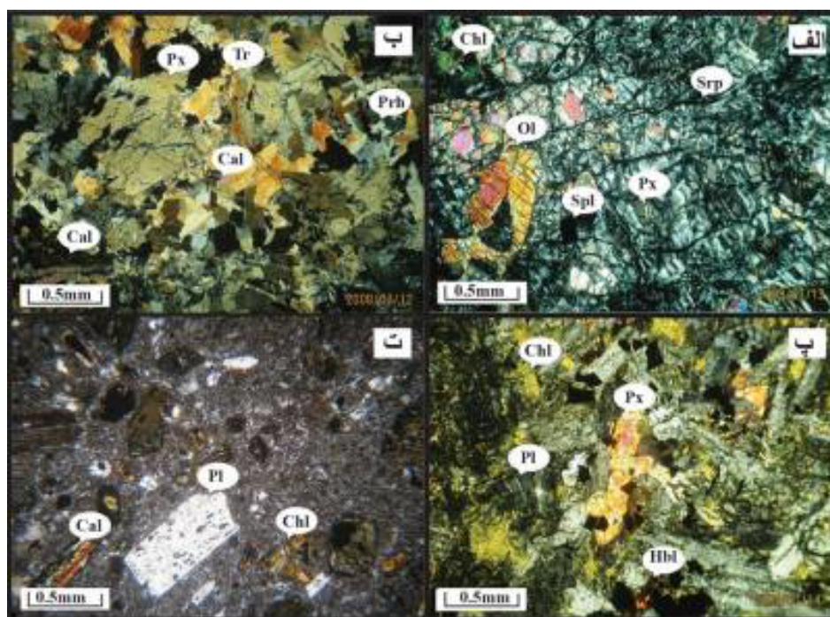
شکل ۳ (الف) بقایایی از اورتوپروکسن که در برخی قسمت‌ها توسط کلریت جانشین شده‌اند به همراه الیون‌های تخم مرغی شکسته شده که توسط سرپانتین جانشین شده‌اند (XPL)، (ب) تره‌مولیت و اکتینولیت که جانشین بلورهای پروکسن شده‌اند، به همراه پره‌نیت که جانشین پلاژیوکلاز شده است و مقادیر اندکی کلسیت (XPL)، (پ) بلورهای پروکسن که در برخی موارد توسط هورنبلند جانشین شده‌اند، به همراه پلاژیوکلاز که به اپیدوت، کلریت و کلسیت دگرسان شده‌اند (XPL)، و (ت) درشت‌بلورهای پلاژیوکلاز که بیشتر آنها به کلسیت و کانی‌های رسی تبدیل شده‌اند، به همراه کلریت در زمینه شیشه‌ای آتشفشانی (XPL). علائم اختصاری بکار رفته عبارتند از: Px= پروکسن، Tr= تره‌مولیت، Cal= کلسیت، Prh= پره‌نیت، Pl= پلاژیوکلاز، Chl= کلریت، Hbl= هورنبلند، Srp= سرپانتین و Ol= الیون. که برگرفته از مرجع [۱۰] هستند.
