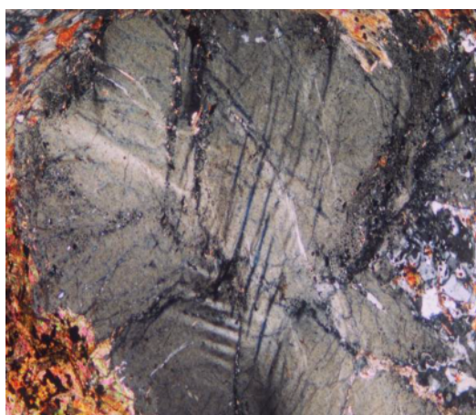
شکل ۱۱ ساختار منطقه‌ای برآمده از دگرشکلی در بلور آندالوزیت (And). عرض عکس برابر با ۴/۲ میلیمتر است.
