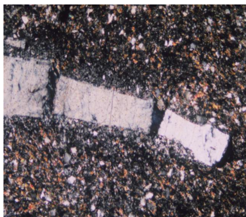
شکل ۱۲ یک بلور کشیده آندالوزیت (And) که دچار شکستگی شده است. عرض عکس برابر با ۳/۲ میلیمتر است.
