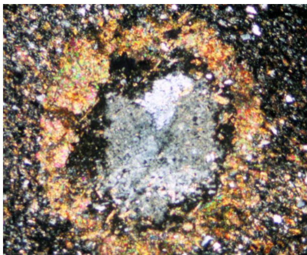
شکل ۲ بقایای کوردیوریت (Crđ) که توسط مجموعه‌های غنی از میکا در حال جایگزینی است. به منطقه‌بندی قطاعی در بلور کوردیوریت توجه نمایید. عرض عکس برابر با ۳/۵ میلیمتر می‌باشد.
