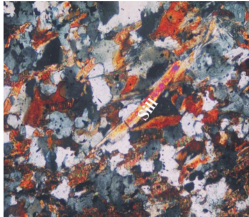
شکل ۶ بلورهای منشوری طویل سیلیمانیت (sill) تشکیل شده در زمینه سنگ. عرض عکس برابر با ۳٫۵ میلیمتر است.
