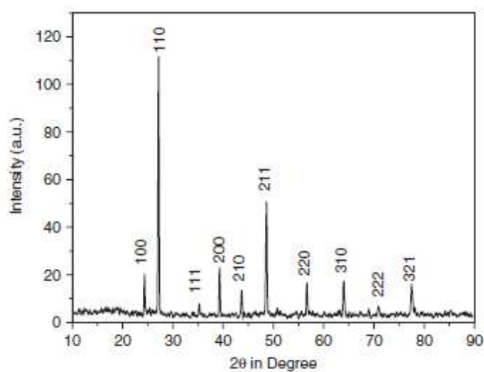
شکل ۵ طیف پراش پرتو ایکس از نمونه CsI.
