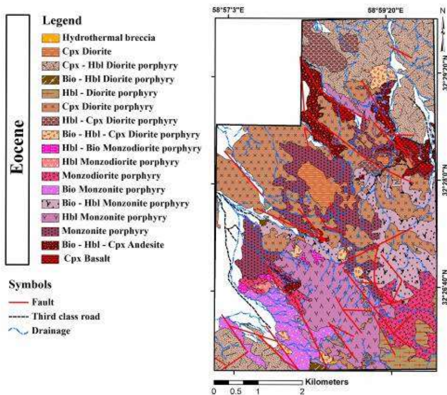
شکل ۲ نقشه زمین‌شناسی گستره شاه سلطان علی با مقیاس ۱:۲۰۰۰۰.
