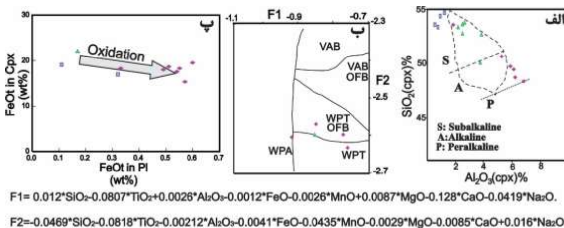
شکل ۷ الف- نمودار SiO 2 نسبت به Al 2 O 3 برای کلینوپیروکسن‌های موجود در دیابازهای سازند هرمز مورد بررسی [۲۹]. ب- نمودار F1-F2 [۳۰] برای کلینوپیروکسن‌های مورد بررسی. VAB: بازالت‌های قوس آتشفشانی؛ VAB OFB: بازالت‌های کف اقیانوسی؛ WPT: بازالت‌های تولیتی درون صفحه‌ای؛ WPA: بازالت‌های قلیایی درون صفحه‌ای. پ- نمودار FeO total در پلاژیوکلاز نسبت به FeO total در کلینوپیروکسن [۳۱] موجود در سنگ‌های دیابازی مورد بررسی. Cpx: کلینوپیروکسن، Pl: پلاژیوکلاز. علائم به کار رفته مشابه شکل ۵ هستند.
