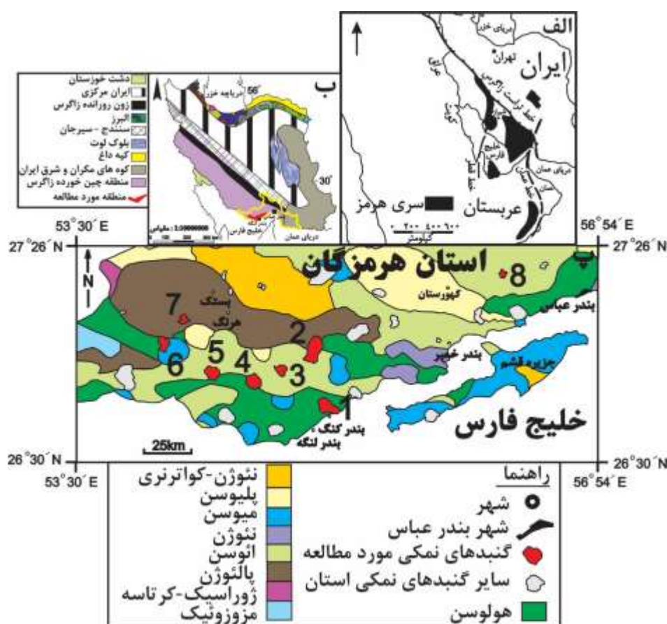
شکل ۱ الف- موقعیت سازند هرمز در ایران و خاورمیانه. وضه رسوبات نمکی جنوب عمان- شمال کرمان دارای روند شمالی- جنوبی بوده و از جنوب عمان، ناحیه هائوشی-هاف تا مرکز ایران کشیده شده است [۲۰]. ب- موقعیت استان هرمزگان در ایران و پهنه‌های ساختاری آن [۲۱]. پ- موقعیت گنبد‌های نمکی مورد بررسی در جنوب ایران (استان هرمزگان). گنبد‌های نمکی ۱: بند معلم، ۲: زندان، ۳: چمپه، ۴: چاه مسلم، ۵: باوردان، ۶: داربست، ۷: گزه و ۸: انگورو [۵].
