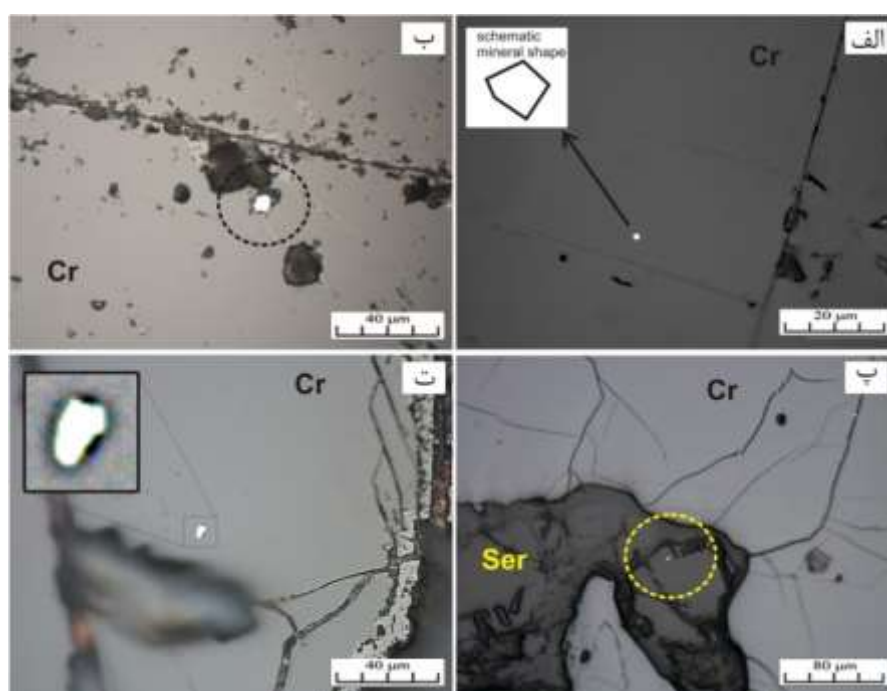
شکل ۴ تصاویر میکروسکوپی کانی‌های احتمالی گروه پلاتین که در بررسی‌های سنگ‌نگاری مشخص شده‌اند: الف) کانی شکل‌دار احتمالی گروه پلاتین در کروم‌اسپینل (Cr) با طرح‌واره‌ای از شکل آن، ب) نمونه شناسایی شده در محل شکستگی کانی کروم‌اسپینل، پ) کانی به دام افتاده در زمینه سیلیکاتی-سرپانتینی (Ser)، و ت) نمونه احتمالی از گروه پلاتین به همراه دو فاز سیلیکاتی (تیره رنگ در تصویر پیوست).
