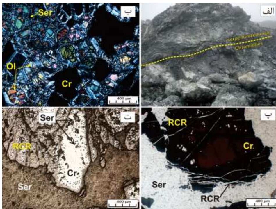
شکل ۲ الف) تصویر صحرایی کرومیت‌های Cr بالا احاطه شده توسط پریدوتیت سرپانتینی شده در بخش غربی افیولیت خوی، ب) الیوین (Ol) و سرپانتین (Ser) در فضای بین دانه‌های کروم اسپینل (Cr)، پ) کروم اسپینل (Cr) به رنگ قهوه‌ای روشن در نور طبیعی عبوری (PPL) و کناره تیره (RCR) به دلیل حضور فروکرومیت از کرومیت‌های Al بالا در بخش شرقی افیولیت خوی، و ت) میانبرهای پر شده با سرپانتین (Ser) در کروم اسپینل.
