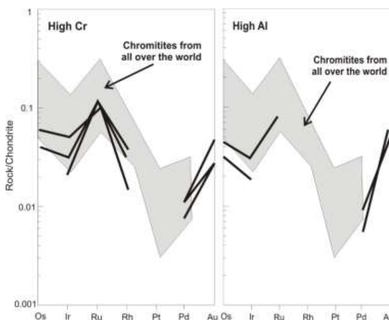
شکل ۵ طرح به هنجار شده عناصر گروه پلاتین و طلا نسبت به کندریت در کرومیتیت‌های غنی از Cr در بخش غربی افیولیت خوی و غنی از Al در بخش شرقی افیولیت خوی (خطوط ممتد) و افیولیت‌های جهان [۵، ۲۴-۱۹].
