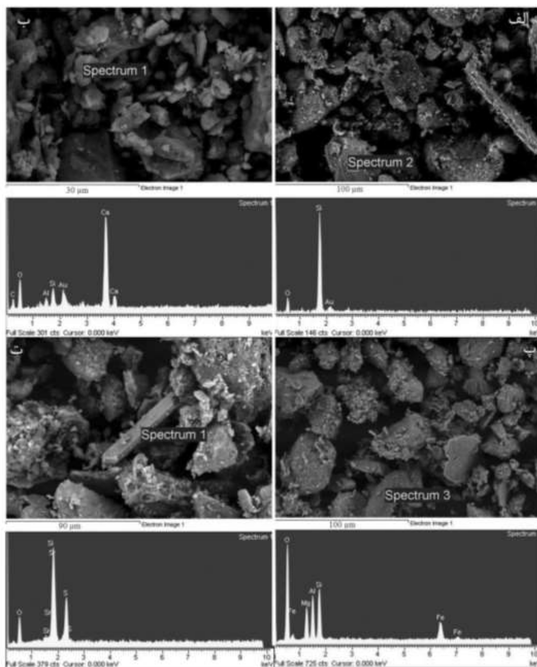
شکل ۵ تصاویر SEM و میکروآنالیز EDX نمونه ریزگردهای گناباد. براساس بررسی‌های EDX فاز کوارتز (شکل الف)، فاز کلسیت (شکل ب)، فاز کانی‌های رسی (ایلیت، شکل پ) و فاز کانی‌های کمیاب (استرونیانیت، شکل ت) بخوبی مشهود است.
