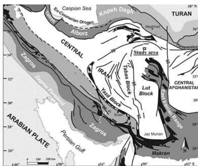
شکل ۱ موقعیت منطقه مورد بررسی و جایگاه آن در پهنه لوت [۱۹].
