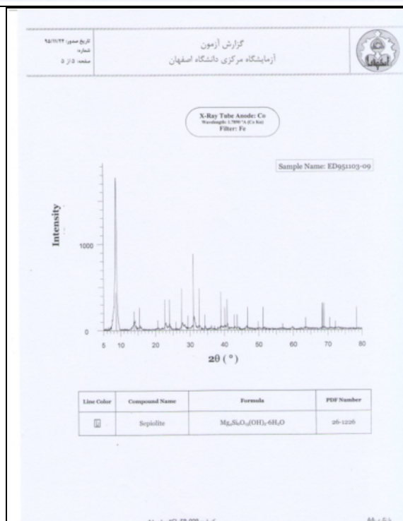
شکل ۴ طیف‌های پراش پرتو X نمونه‌های مورد بررسی که نشان دهنده حضور سپیولیت در آنهاست، الف- نمونه ناخالص سپیولیت در سنگ میزبان لیستونی، ب- نمونه خالص سپیولیت رشته‌ای و پ- نمونه خالص سپیولیت توده‌ای.
