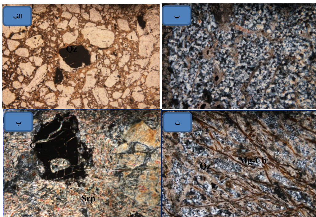
شکل ۳ الف: بافت ریزدانه‌ای و ب: بافت تنش آواری در لیستونیت‌ها، پ: حضور کروم اسپینل در لیستونیت‌ها، ت: بقایای بافت سرپانتینیت پس از لیستونیتی شدن، تصاویر میکروسکوپی در نور قطبشی با پهنای دید ۳ میلیمتر برداشت شده‌اند (Chr = کرومیت، Srp = سرپانتین، Qz = کوارتز، Mg-Cb = کربنات‌های منیزیم‌دار، علائم اختصاری برگرفته از مرجع [۱۳] هستند).
