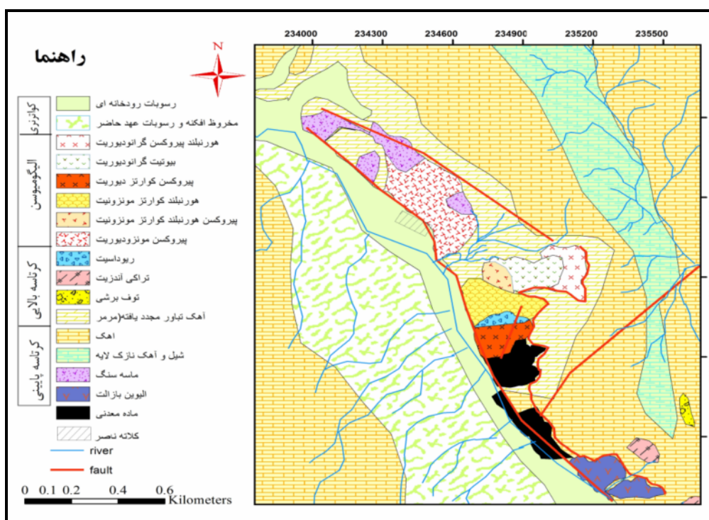
شکل ۱ الف) نقشه تقسیمات ساختمانی ایران [۱۵] که موقعیت منطقه مورد بررسی با علامت ستاره بر آن مشخص شده است و (ب) نقشه زمین‌شناسی منطقه مورد بررسی.
