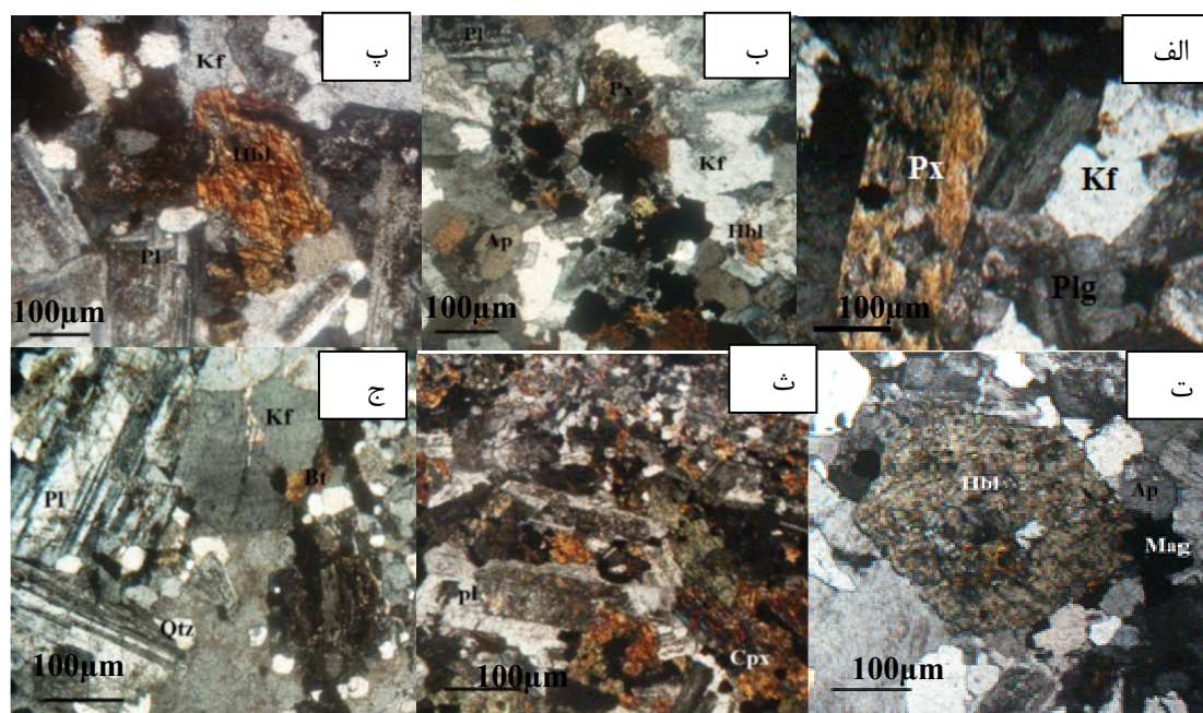
شکل ۲ تصاویر میکروسکوپی از توده های نفوذی منطقه الف) پیروکسن مونزودیوریت، ب) پیروکسن هورنبلند کوارتز مونزونیت، پ) هورنبلند کوارتز مونزونیت، ت) پیروکسن کوارتز دیوریت، ث) بیوتیت گرانودیوریت، ج) هورنبلند پیروکسن گرانودیوریت، نور XPL. (علائم اختصاری برگرفته از مرجع [۱۸]).
