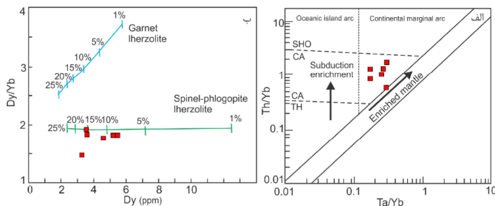
شکل ۸ الف) موقعیت توده‌های نفوذی جلمبادان در نمودار Th/Yb نسبت به Ta/Yb [۲۴]، TH = تولیتی، CA = آهک-قلیایی، SHO = شوشونیتی ب) نمودار Dy/Yb نسبت به Dy [۳۱] برای تعیین خاستگاه توده‌ها.
